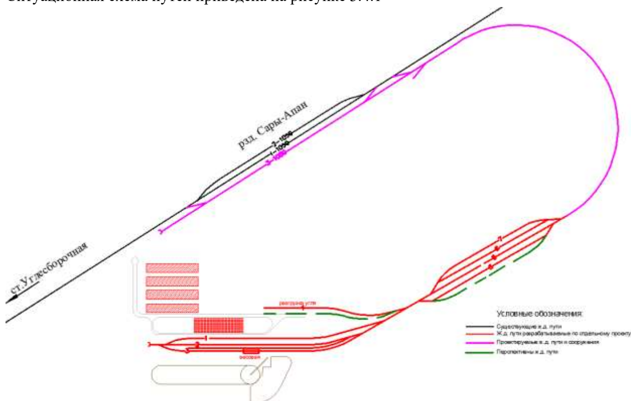
Рисунок 3.4.1 Схема станции Заводская
