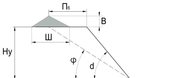
Рис.3.4.1 Схема уступа
