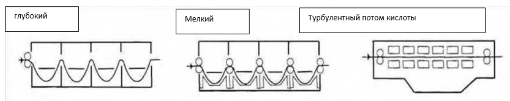
Рисунок 5.2 - Различные типы ванн травления
