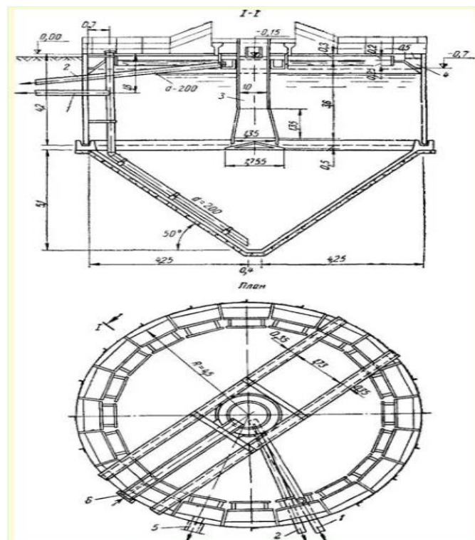
Рисунок 5.24 - Конструкция вертикального отстойника
