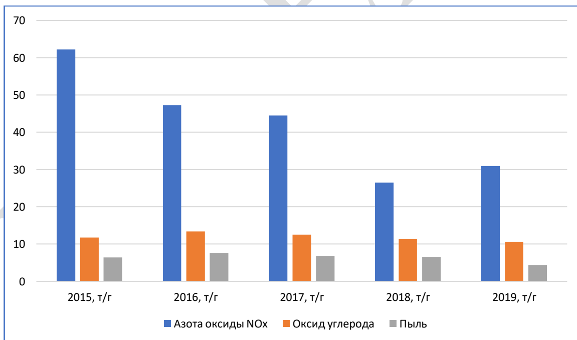
Рис.1.8 - Выбросы и удельные показатели ЗВ за 2015-2019 гг. (при нанесении покрытий на трубы (эпоксидное, полиэтиленовое, полипропиленовое, цинковое))
