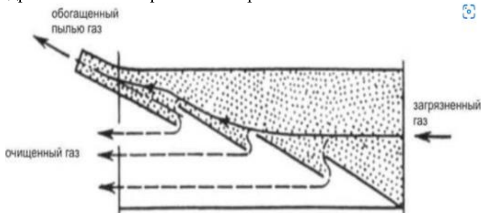
Рисунок 5.10 - Жалюзийный пылеотделитель
