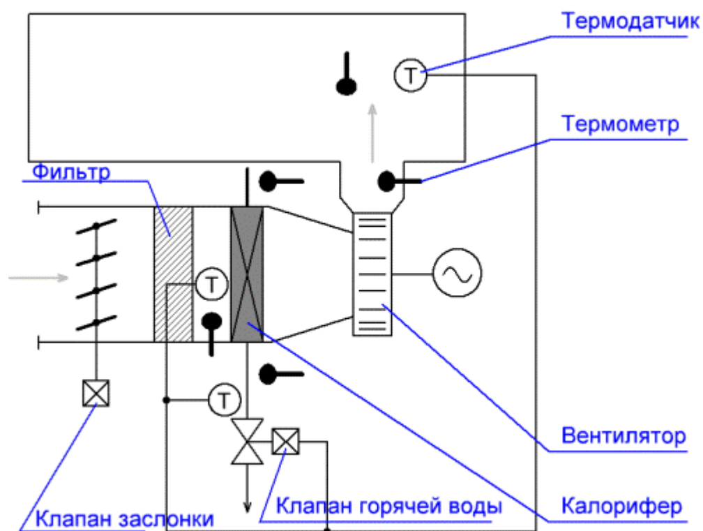
Рисунок 5.1. - Пример автоматической регулировки в системе вентиляции
