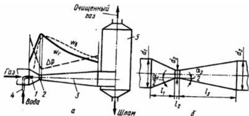
1-конфузор, 2-горловина, 3-диффузор, 4-подача воды, 5-каплеуловитель; а-общий вид, б-нормализованная труба Вентури
