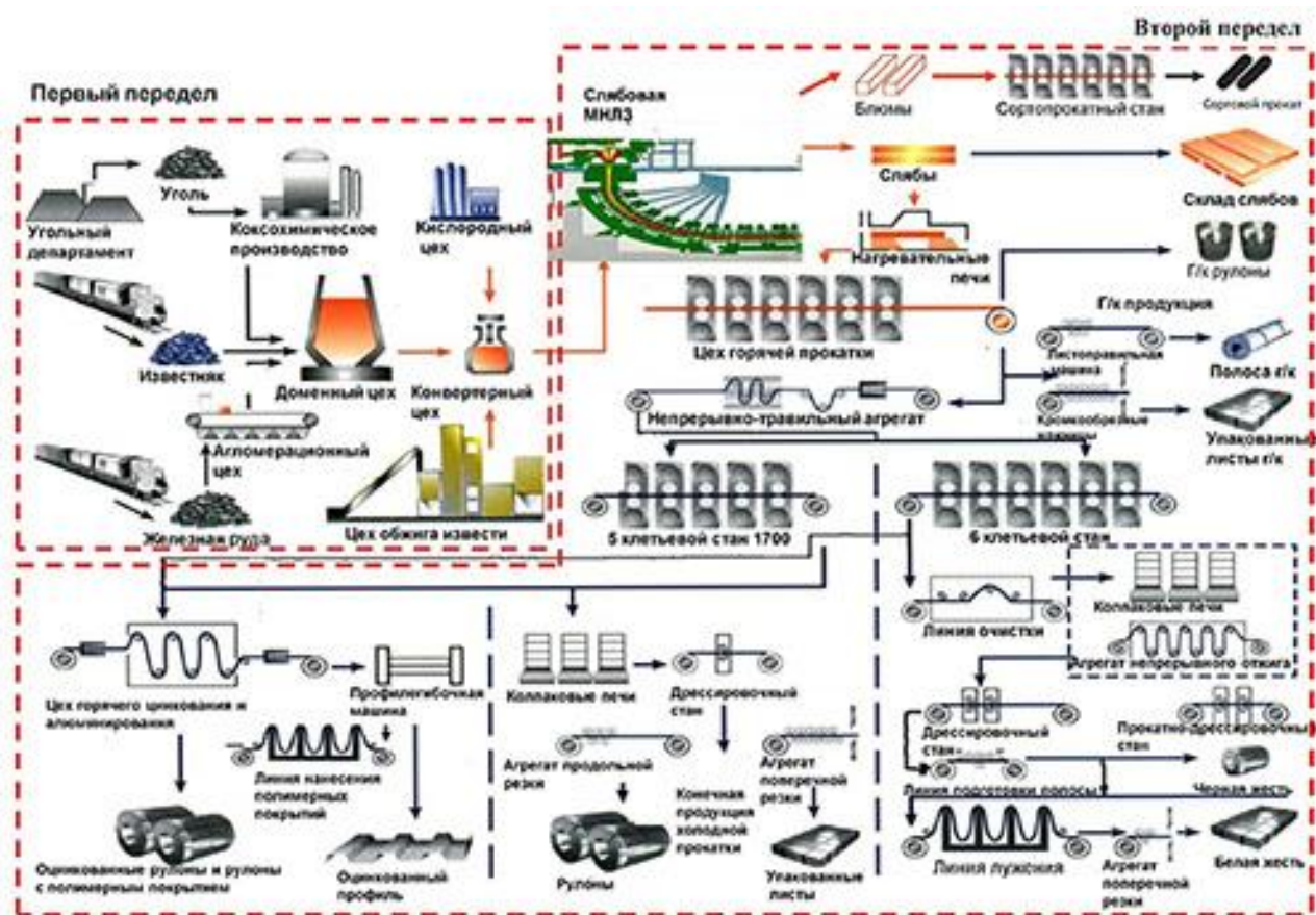
Рисунок 1.1 - Общая схема производства стального департамента АО «АрселорМиттал Темиртау»
