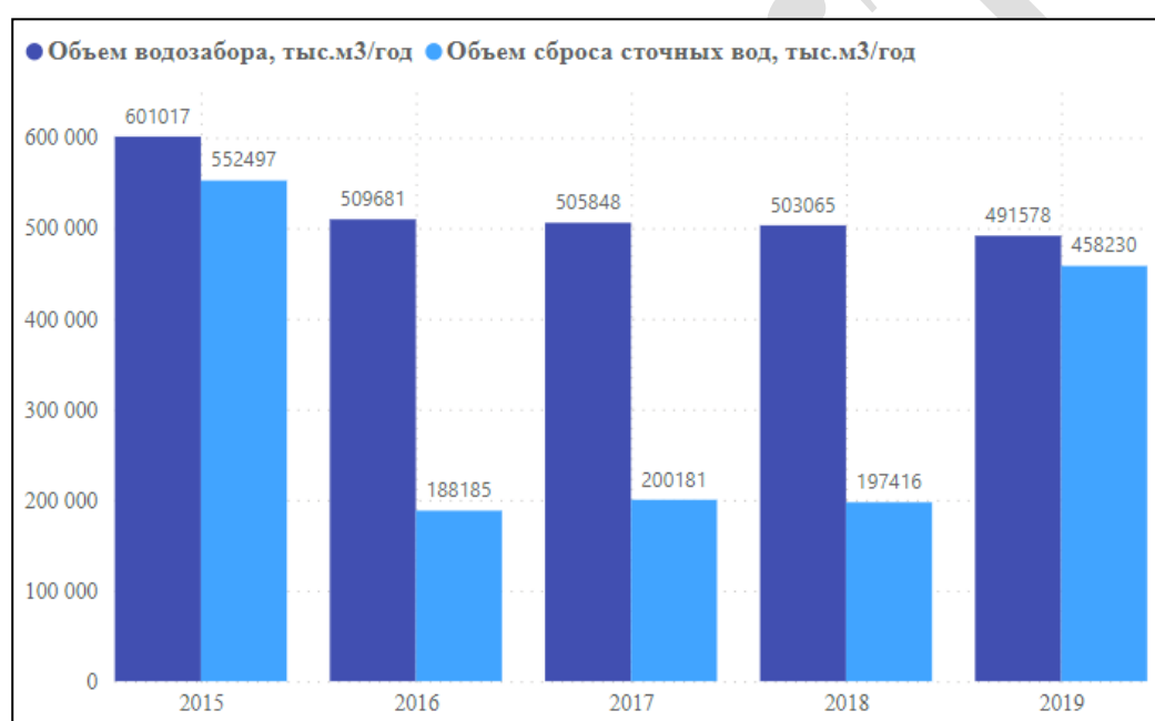
Рис.1.11 - Объемы водопотребления и водоотведения за период с 2015 по 2019 года по предприятию А
