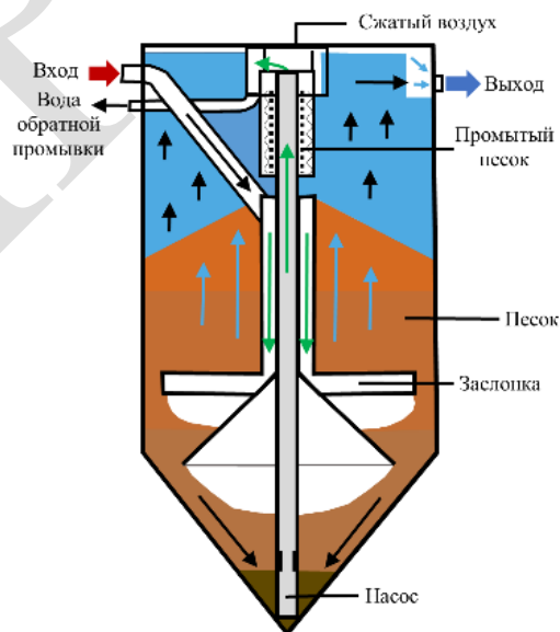
Рисунок 5.25 - Схема песчаного фильтра
