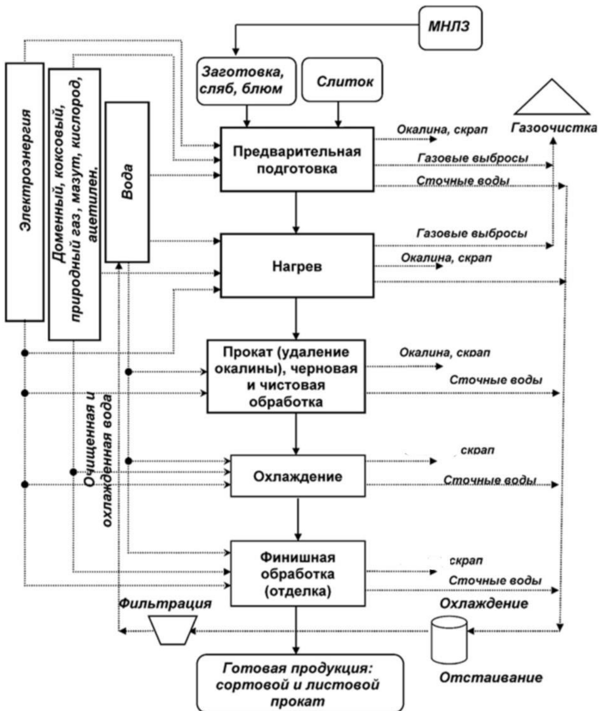
Рисунок 3.1 – Обобщенная технологическая схема производства горячекатаного проката
