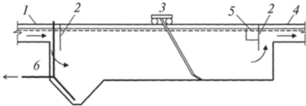
1 — подводящий лоток; 2 — полупогружная доска; 3 — скребковая тележка; 4 — отводящий лоток; 5 — жиросборный лоток; 6 — удаление осадка
