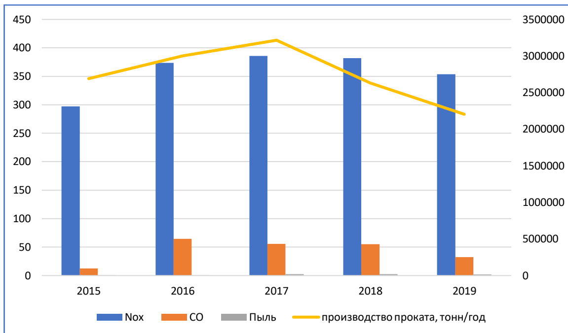
Рис.1.5 - Выбросы и удельные показатели ЗВ за 2015-2019 гг. (от производства горячекатаного плоского проката).
