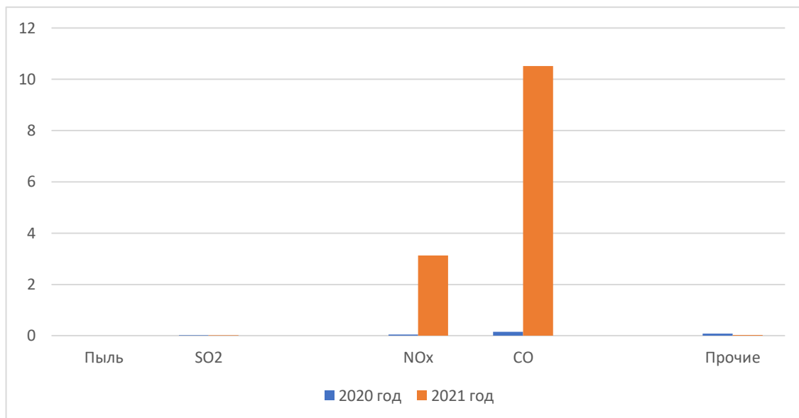
Рис.1.9 - Выбросы ЗВ Предприятия В за 2020-2021 гг. (при производстве горячекатаного проката/шаропроката)
