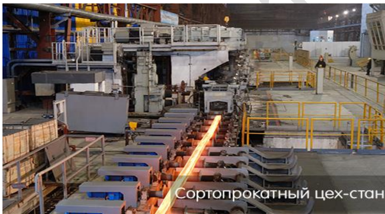
Рисунок 3.3 - Сортопрокатный стан
