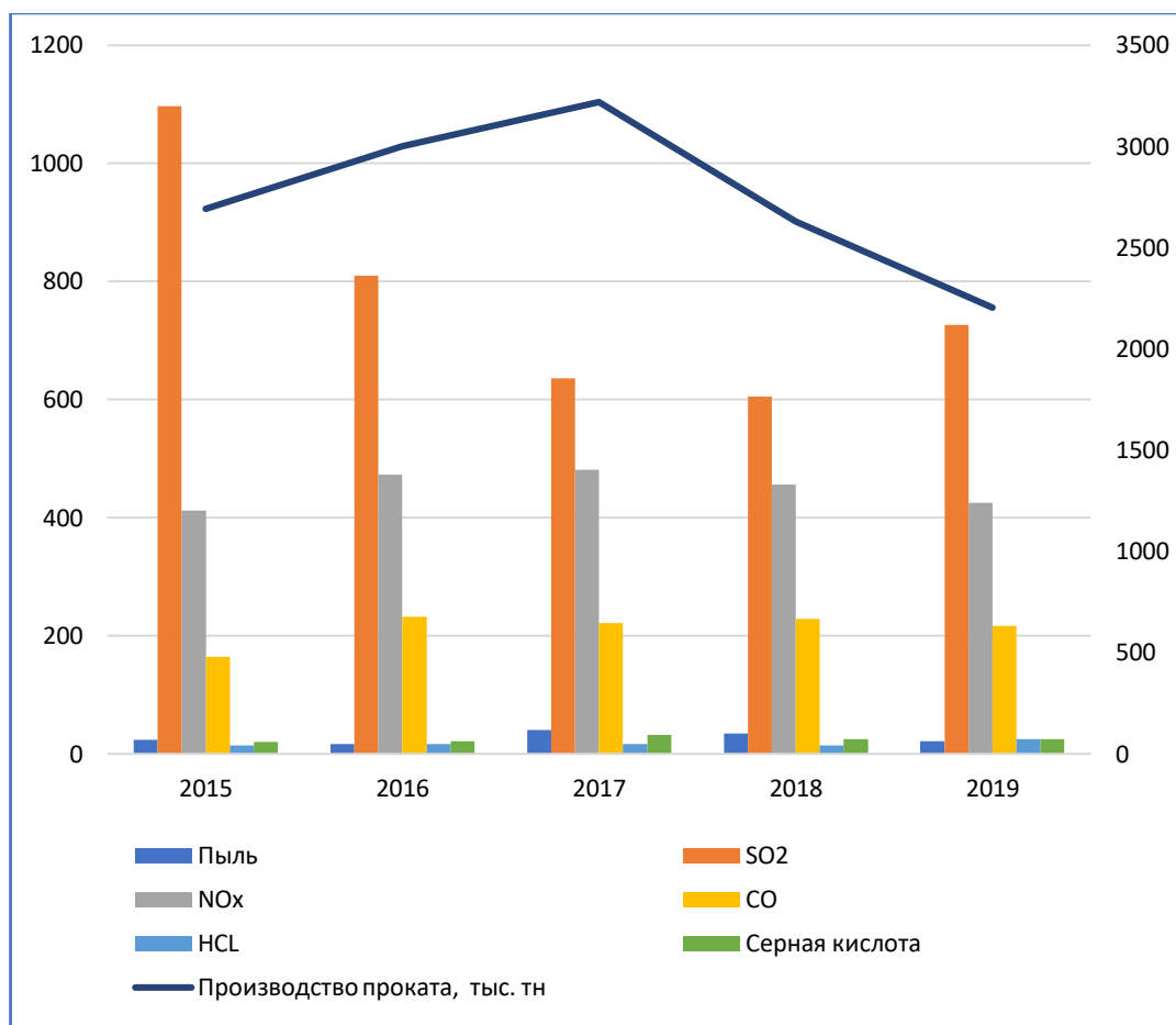
Рис.1.4 - Выбросы и удельные показатели ЗВ за 2015–2019 гг. (общие по прокатному производству).
