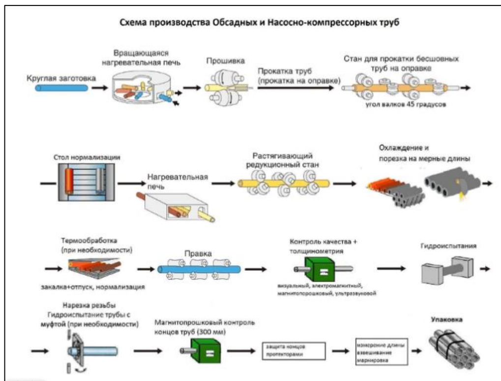
Рисунок 3.16 - Схема производства обсадных и насосно-компрессорных труб
