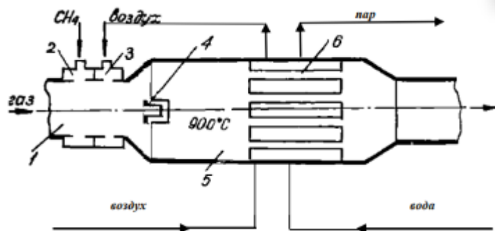
1 – газоход; 2,3 – патрубок; 4 – запальная свеча; 5 - камера дожигания; 6 – теплообменный утилизатор
