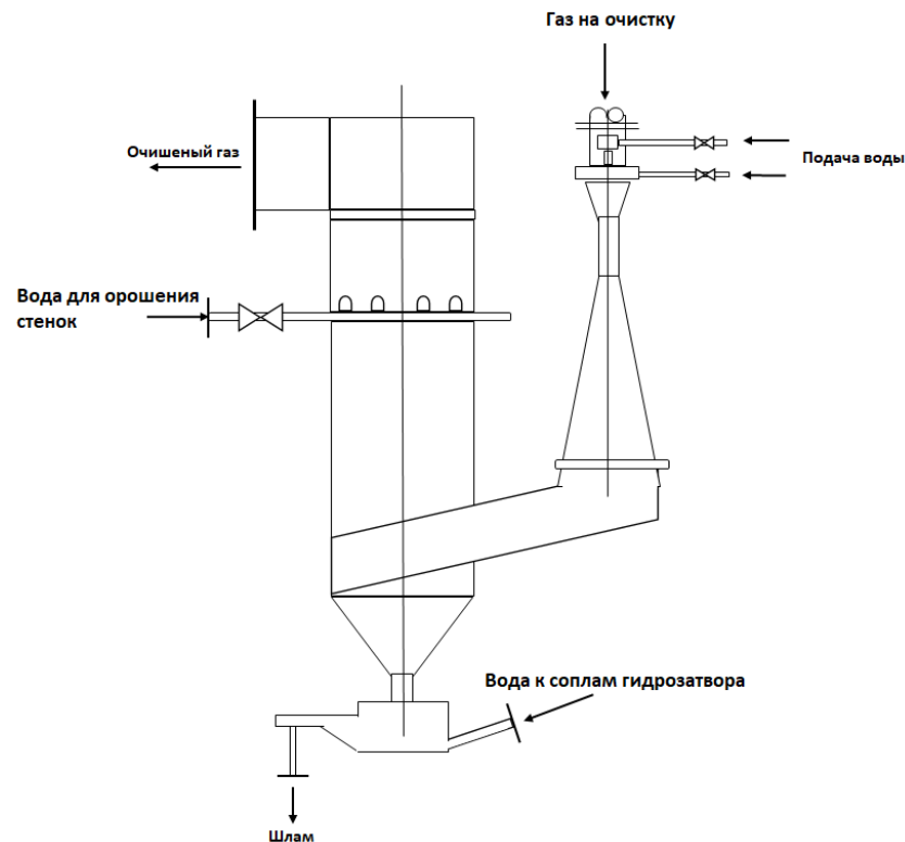
Рисунок 5.14 - Радиальный мокрый скруббер
