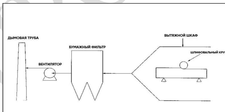
Рисунок 5.4 - Технологическая схема с предотвращением загрязнением в процессе зачистки
