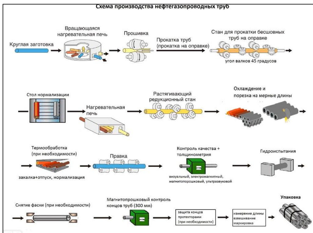
Рисунок 3.15 - Схема производства нефтегазопроводных труб
