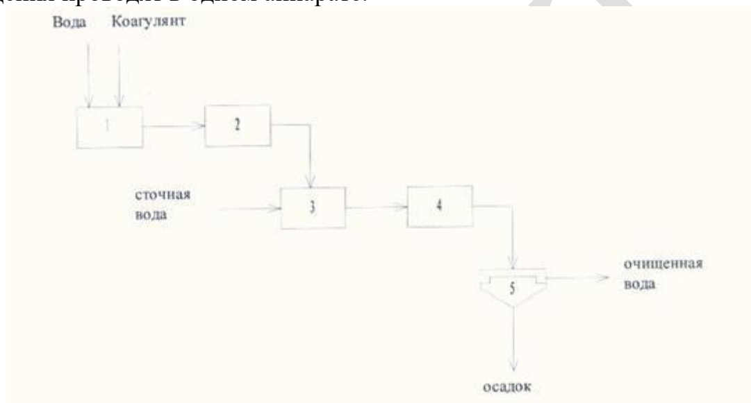
Рисунок 5.26 - Схема процессов коагуляции и флокуляции
