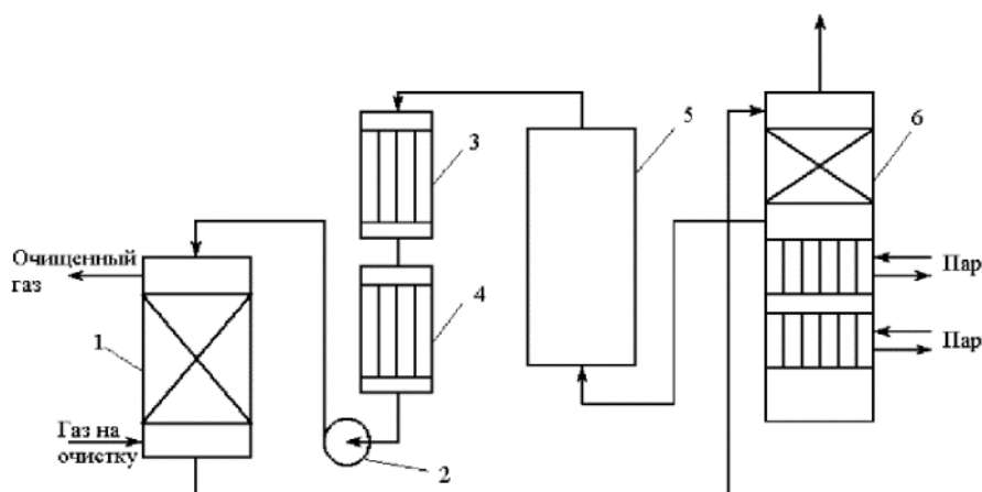
1 - абсорбер; 2 - насос; 3 - водяной холодильник; 4 — аммиачный холодильник 5 - емкость; 6 – десорбер
