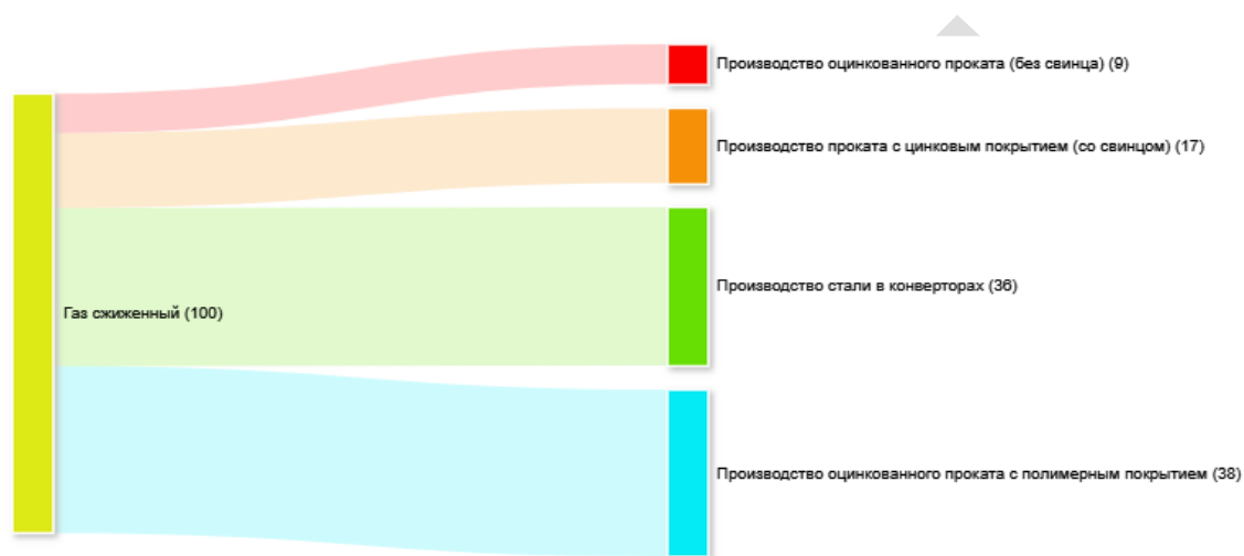
Рисунок 1.3 - Потребление сжиженного газа.
