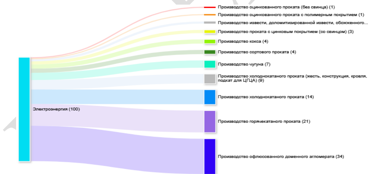
Рисунок 1.2 - Потребление электроэнергии по технологиям производства
