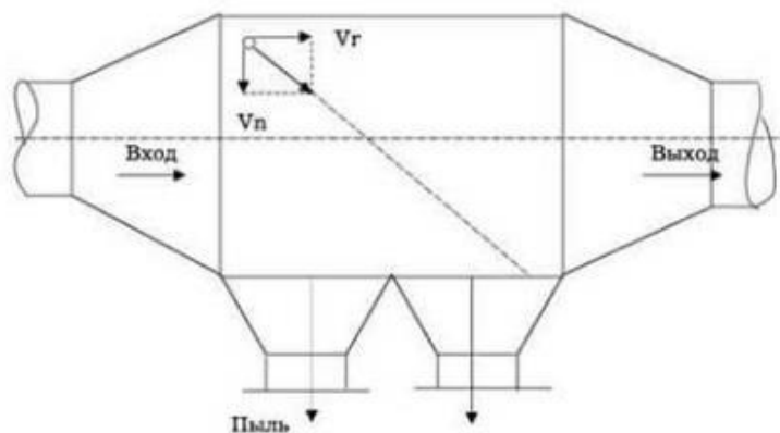
Рисунок 5.9 - Схема горизонтальной осадительной системы
