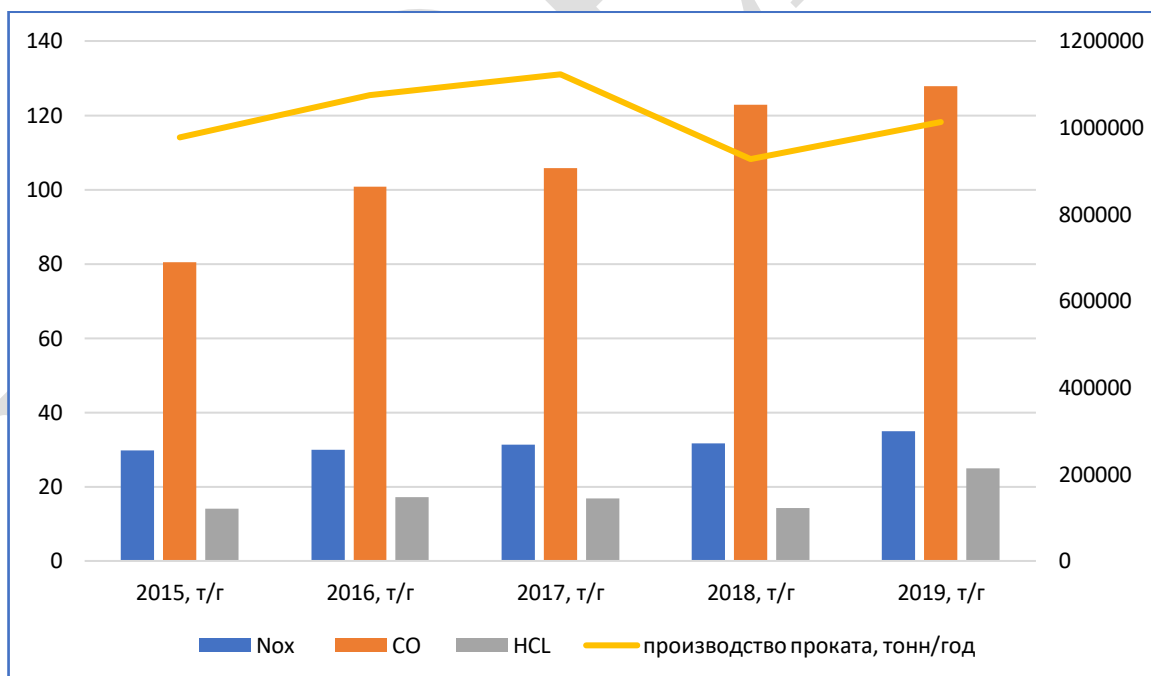
Рис.1.6 - Выбросы и удельные показатели ЗВ за 2015-2019 гг. (от производства холоднокатаного плоского проката).
