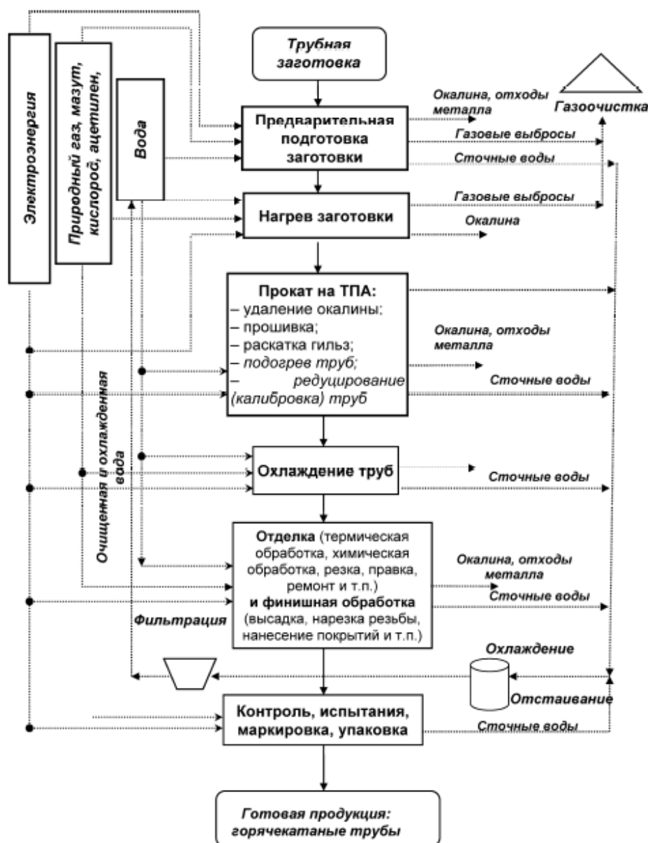
Рисунок 3.13 - Общая схема технологических операций при производстве горячекатаных труб
