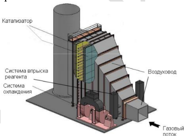
Рисунок 5.18 - Схематичное изображение системы СКВ
