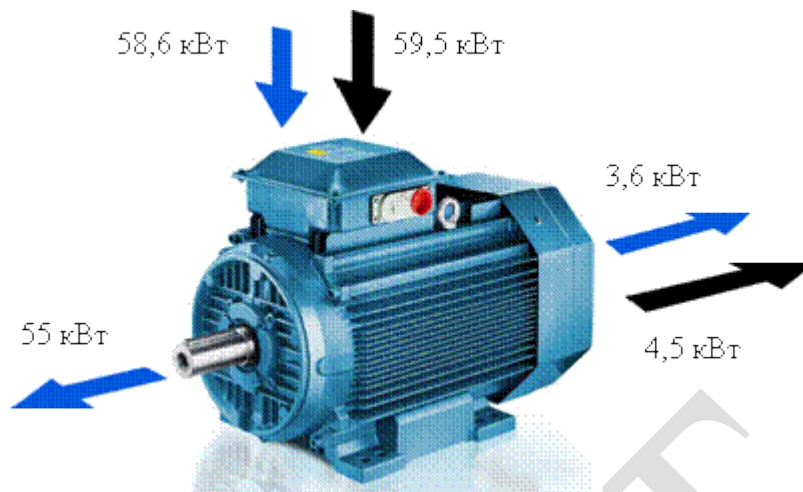
Рисунок 5.5 - Сравнение обычного электродвигателя с энергоэффективным
