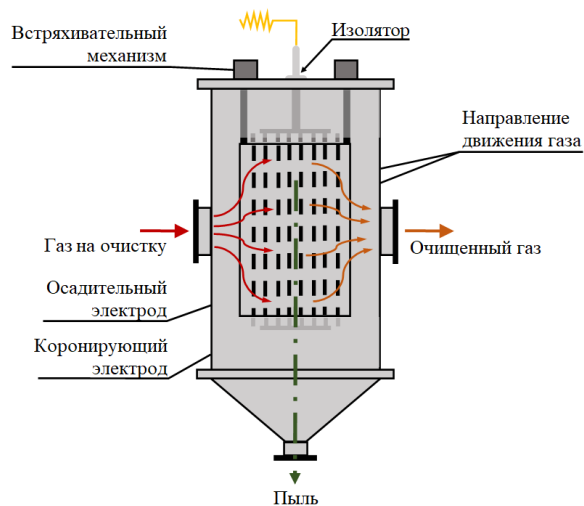
Рисунок 5.12 - Схема устройства электрофильтра (показаны только две зоны)
