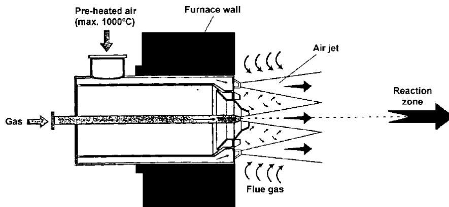
Рисунок 5.16 - Схема горелки с низким содержанием \text{NO}_x и внутренней рециркуляцией дымовых газов
