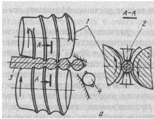
a — в двухвалковом стане; 1 — валки; 2 — направляющие линейки; 3 — исходная заготовка; 4 — заготовка шара
