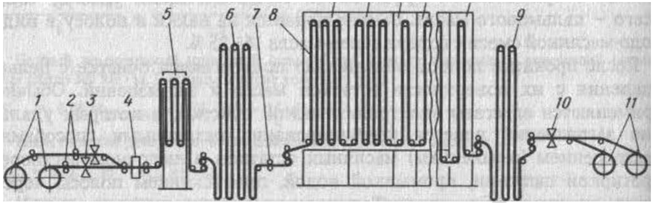
1 — разматыватели; 2 — тянущие ролики; 3 — ножницы; 4 — машина для сварки концов полос; 5 — установка очистки полосы; 6, 9 — накопители полосы (петлевые башни); 7 — дисковые ножницы для обрезки боковых кромок; 8 — отжигательная печь (камеры: а — нагрева; б — выдержки; в — замедленного охлаждения; з — ускоренного охлаждения; д — окончательного охлаждения); 10 — ножницы для вырезки мест сварки; 11 — моталки
