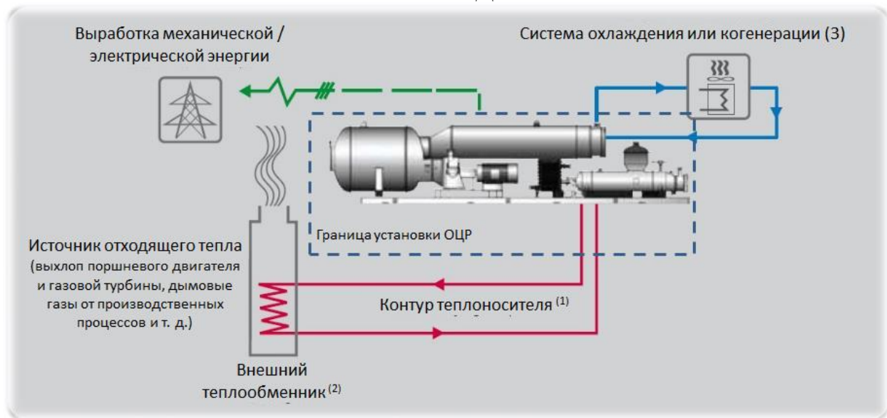
Рисунок 7.1 - Принципиальная схема органического цикла Ренкина
