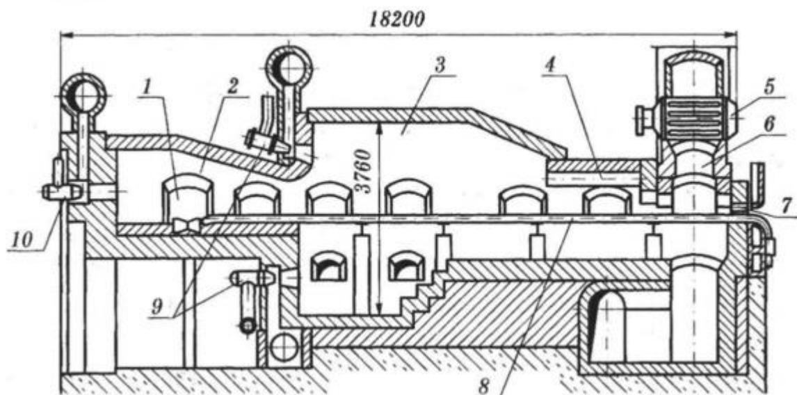
1 — окно для выталкивания заготовок; 2 — сварочная зона; 3 — зона методического нагрева; 4 — зона подогрева; 5 — рекуператоры; 6 — газовые каналы; 7 — посадочное окно (для заготовок); 8 — глиссажные трубы; 9, 10 — газовые горелки
