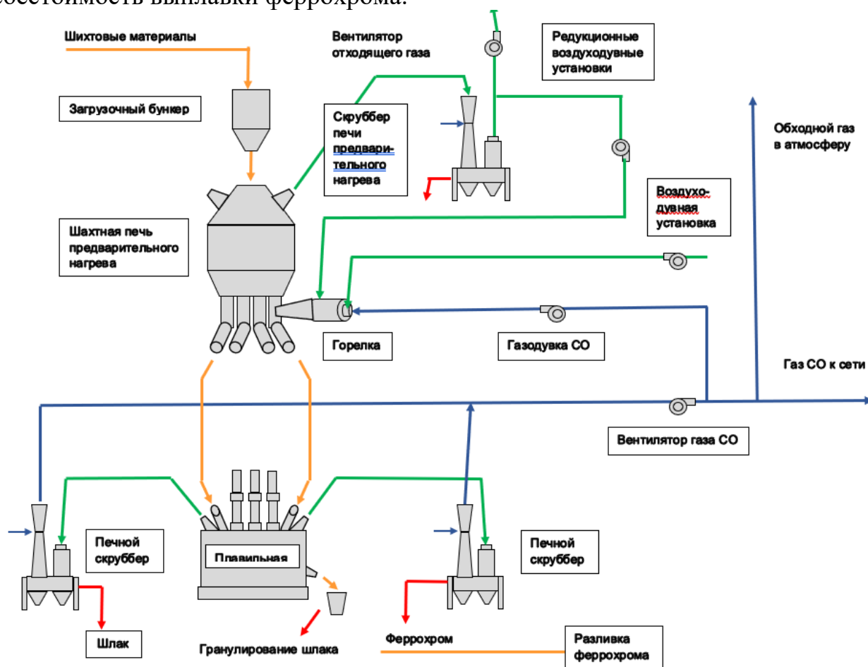
Рисунок 7.6.1 Технологическая схема предварительного нагрева, плавки и газоочистки в процессе производства феррохрома (компания Outotec)
