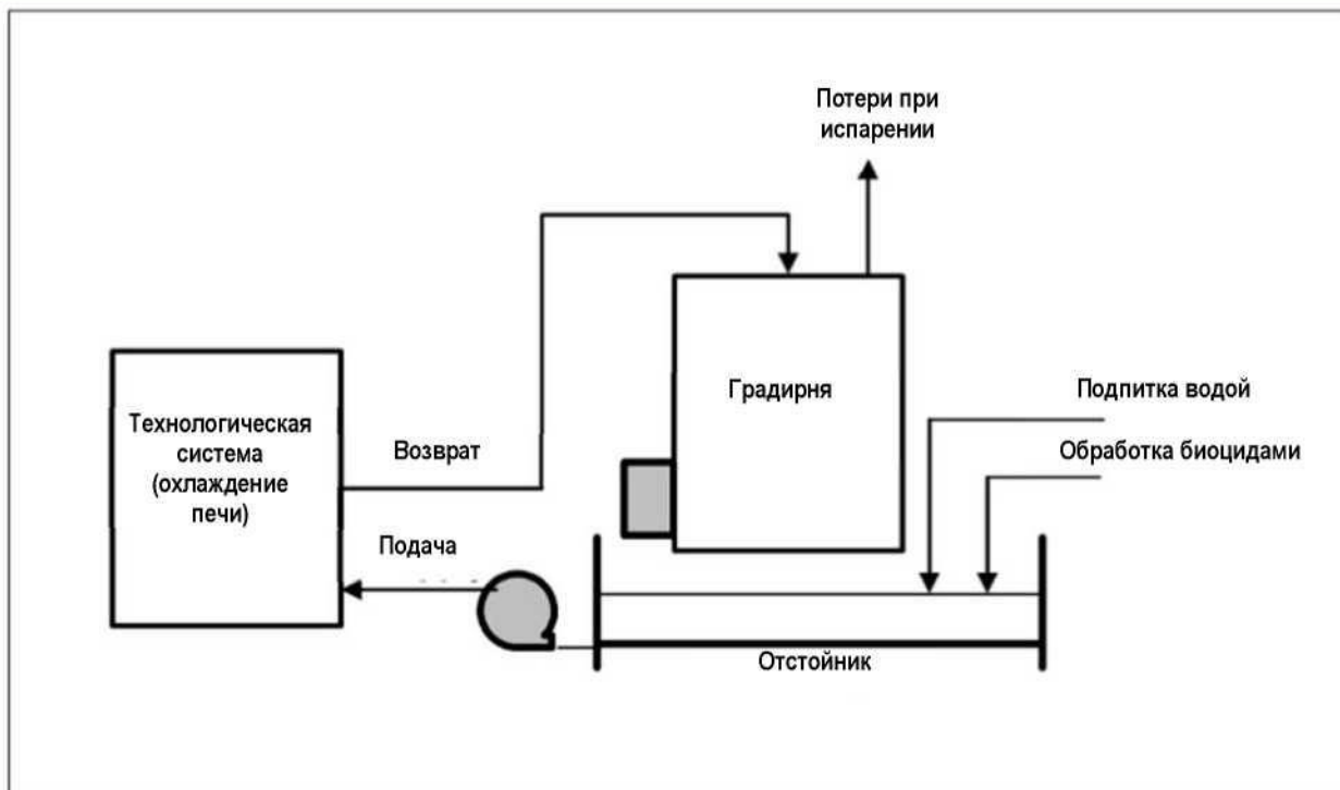
Рисунок 4.9.1 Пример системы рециркуляции воды для охлаждения
