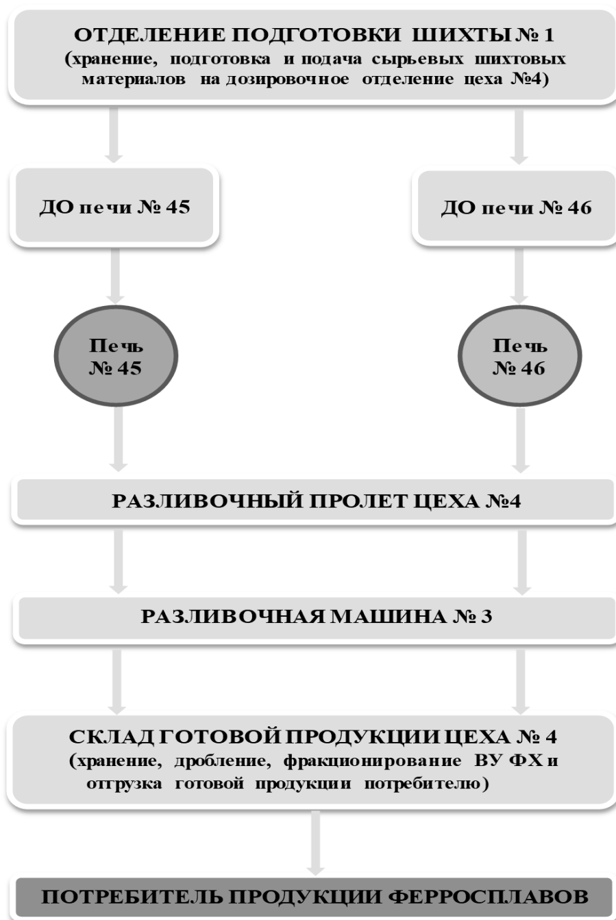
Рисунок 3.1.2.1 Технологическая схема производства ферросилиция
