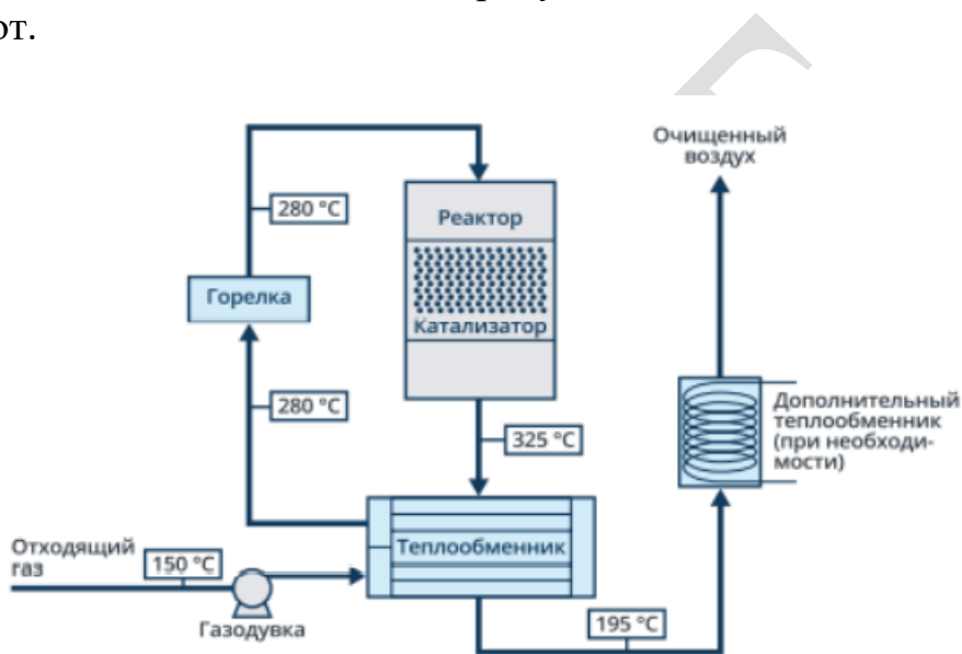
Рисунок 7.7.1 Принципиальная схема САТОХ
