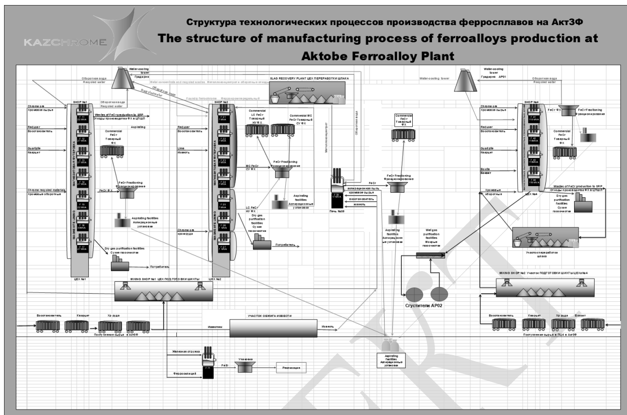
Рисунок 3.1.2.3 Структура технологических процессов производства ферросплавов на АктЗФ
