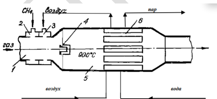
Рисунок 5.7.3 Некаталитическое дожигание СО
