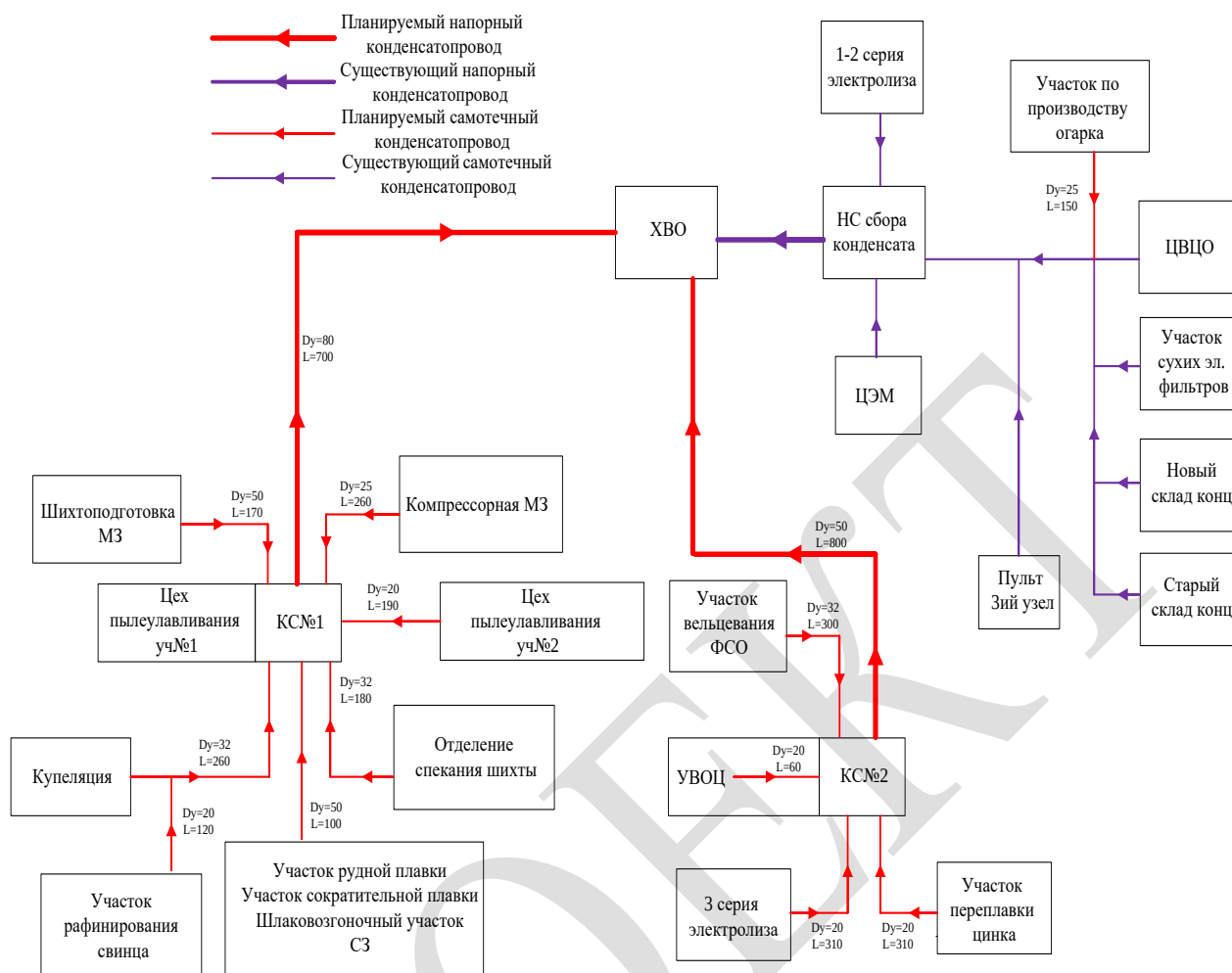
Рисунок 7.2.1 Принципиальная Схема системы возврата конденсата
