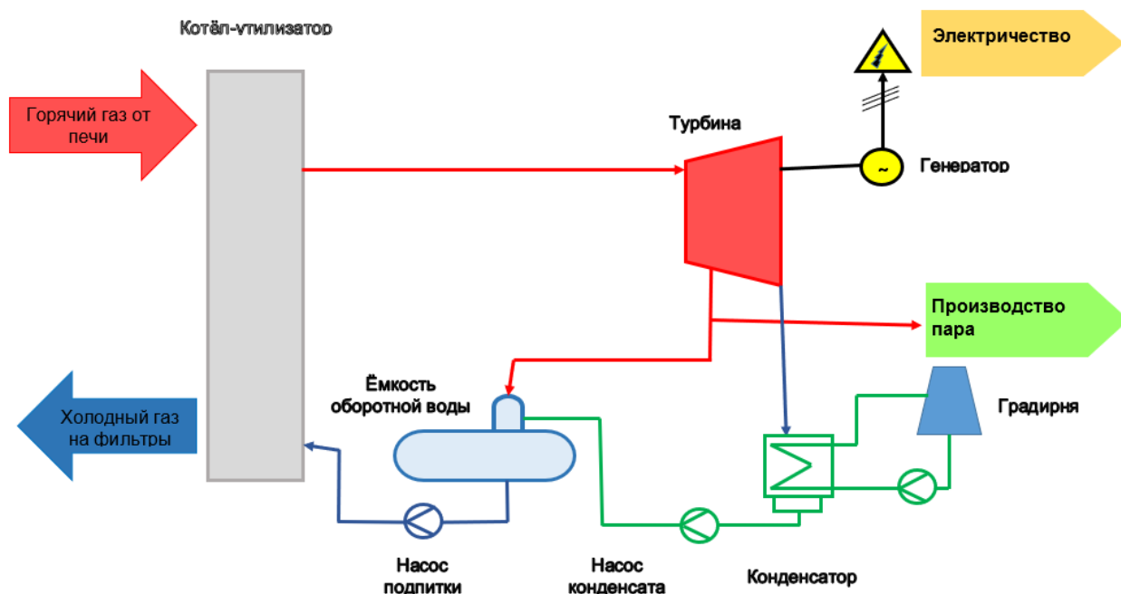
Рисунок 5.1 Типичная блок-схема рекуперации энергии от руднотермической печи
