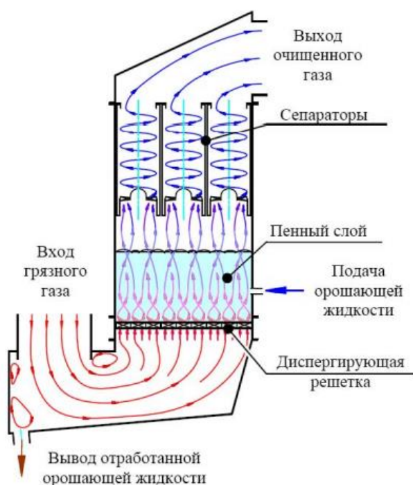
Рисунок 7.8.1 Схема устройства МВГ
