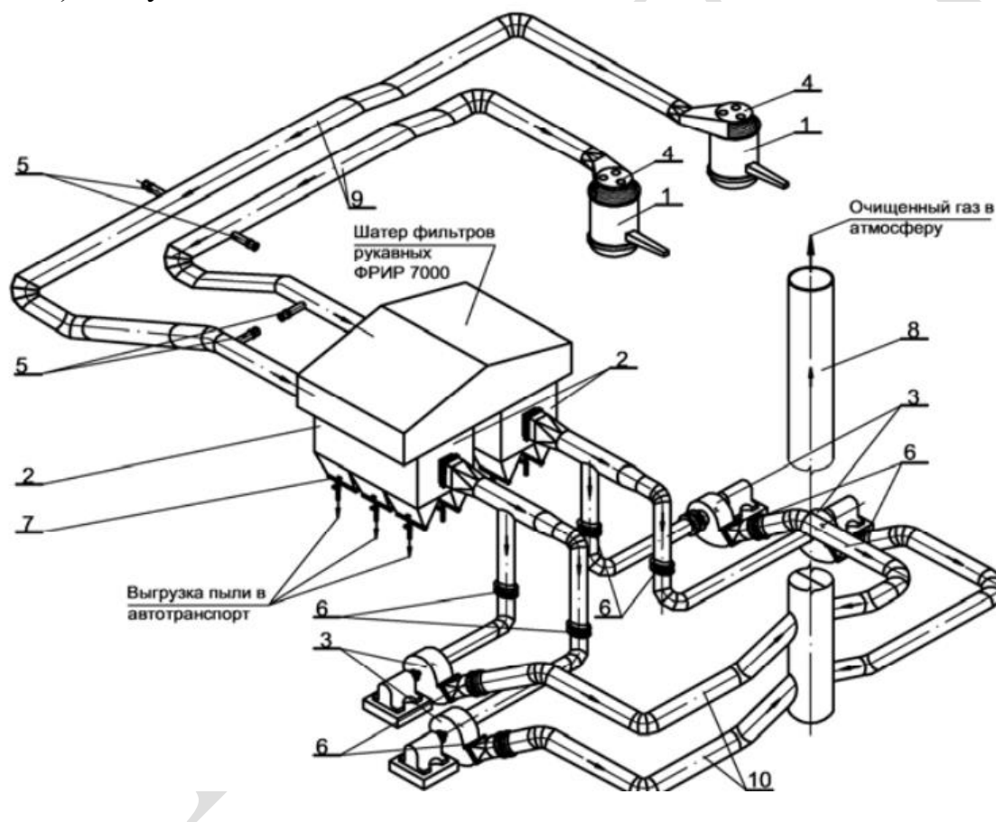
Рис. 5.2. Схема газоочистки открытых ферросплавных печей РКО-25 в цехе № 3 ТОО «Таразский металлургический завод»:
