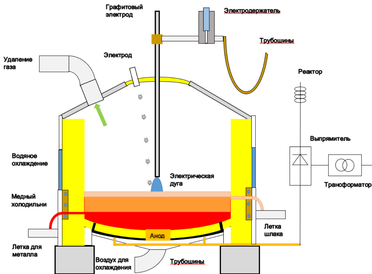
Рисунок 7.6.2 Принципиальная схема печи постоянного тока
