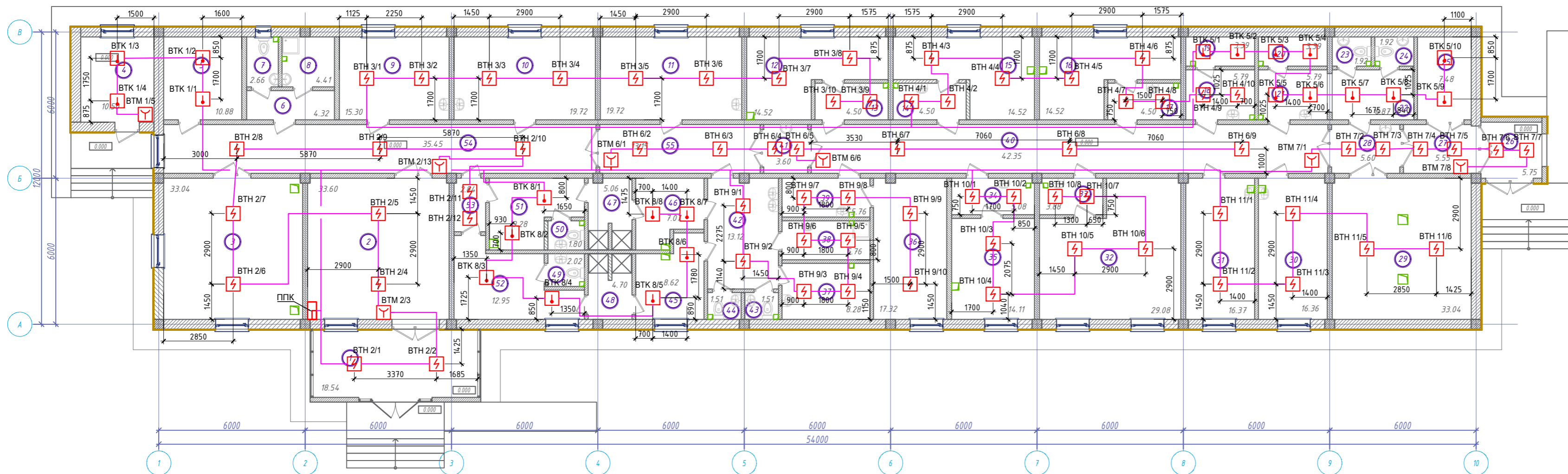
План этажа на отметке 0.000
