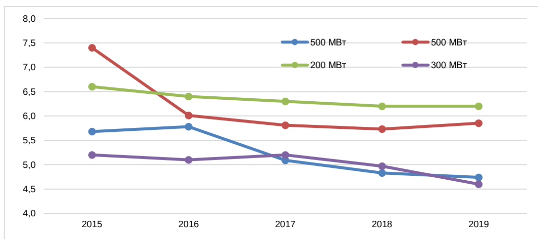
Рис.1.30 – Энергоемкость угольных ТЭЦ 140 кг/см 2 , тут/млн.тенге (по данным КТА МЦЗТуИП)
