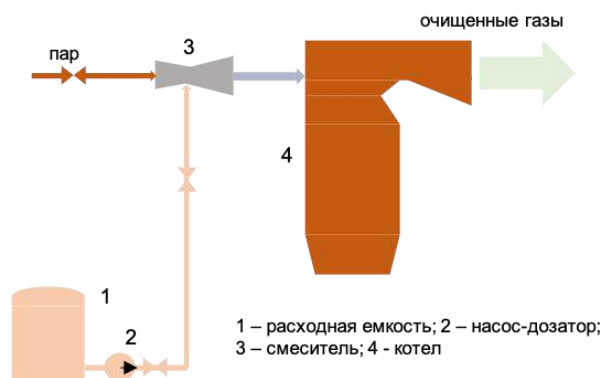
Рис.5.41 – Схема СНКВ
