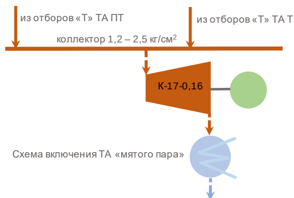
Рис.5.59 – Схема включения турбины «мятого» пара
