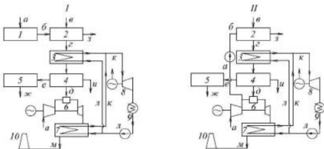
Рис. 7.2 - Принципиальные схемы ПГУ
