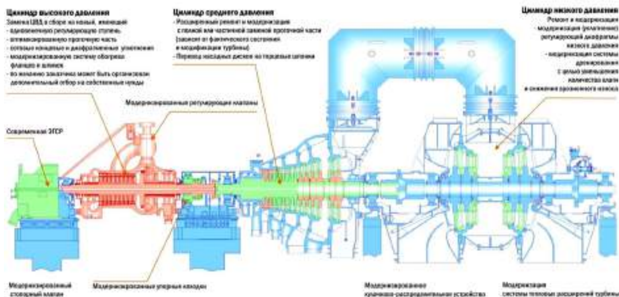
Рис.5.57 – Схема реконструкции Т-100-130
