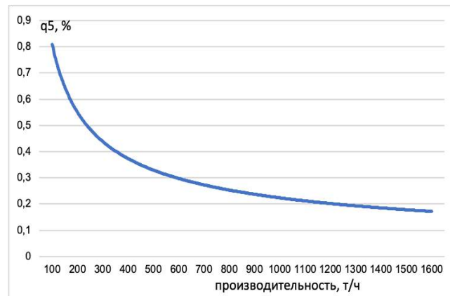
Рис.3.2 – Потеря тепла от наружного охлаждения
