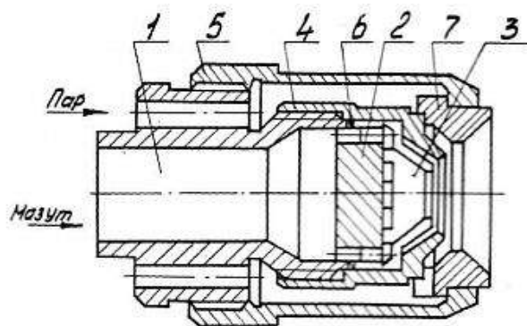
Рис.5.34 – Паромеханическая мазутная форсунка
