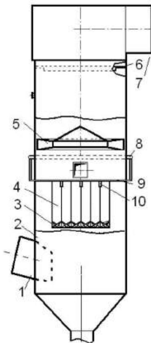
Рис. 4.7 - Схема батарейного эмульгатора второго поколения
