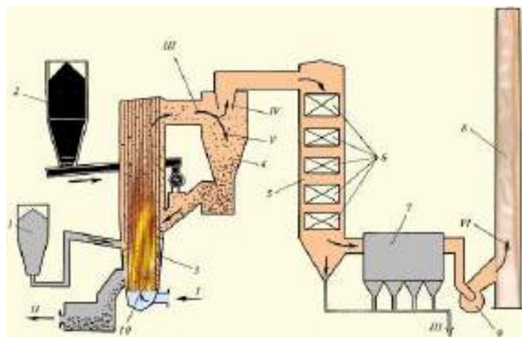
Рис. 5.5 - Принципиальная технологическая схема котла ЦКС
