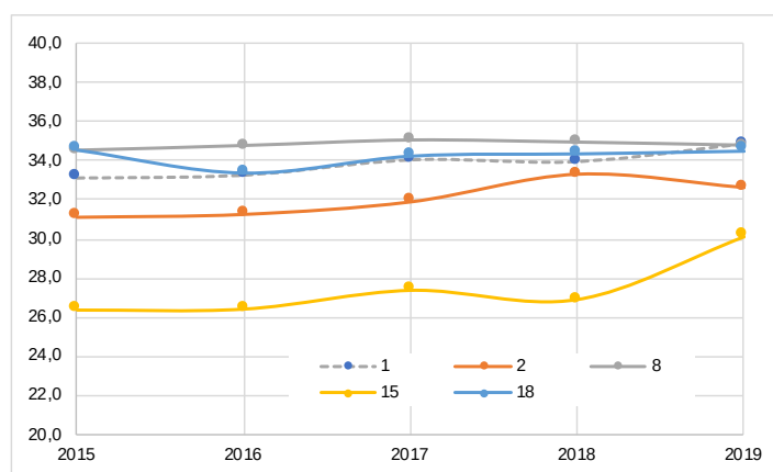
Рис.1.11 – Электрический КПД КЭС, %
