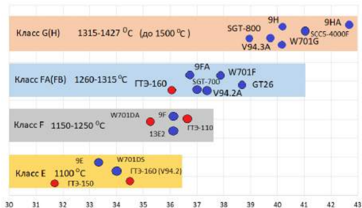
Рис. 3.6 - Показатели эффективности ГТУ в зависимости от температуры газов на входе в газовую турбину
