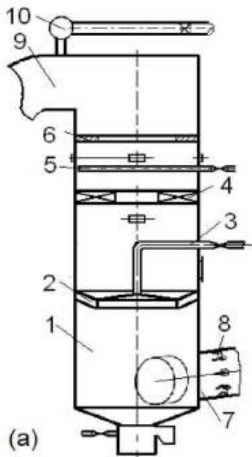
Рис. 4.8 - Кольцевой эмульгатор
