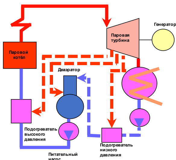
Рис.3.1 – Принципиальная схема КЭС
