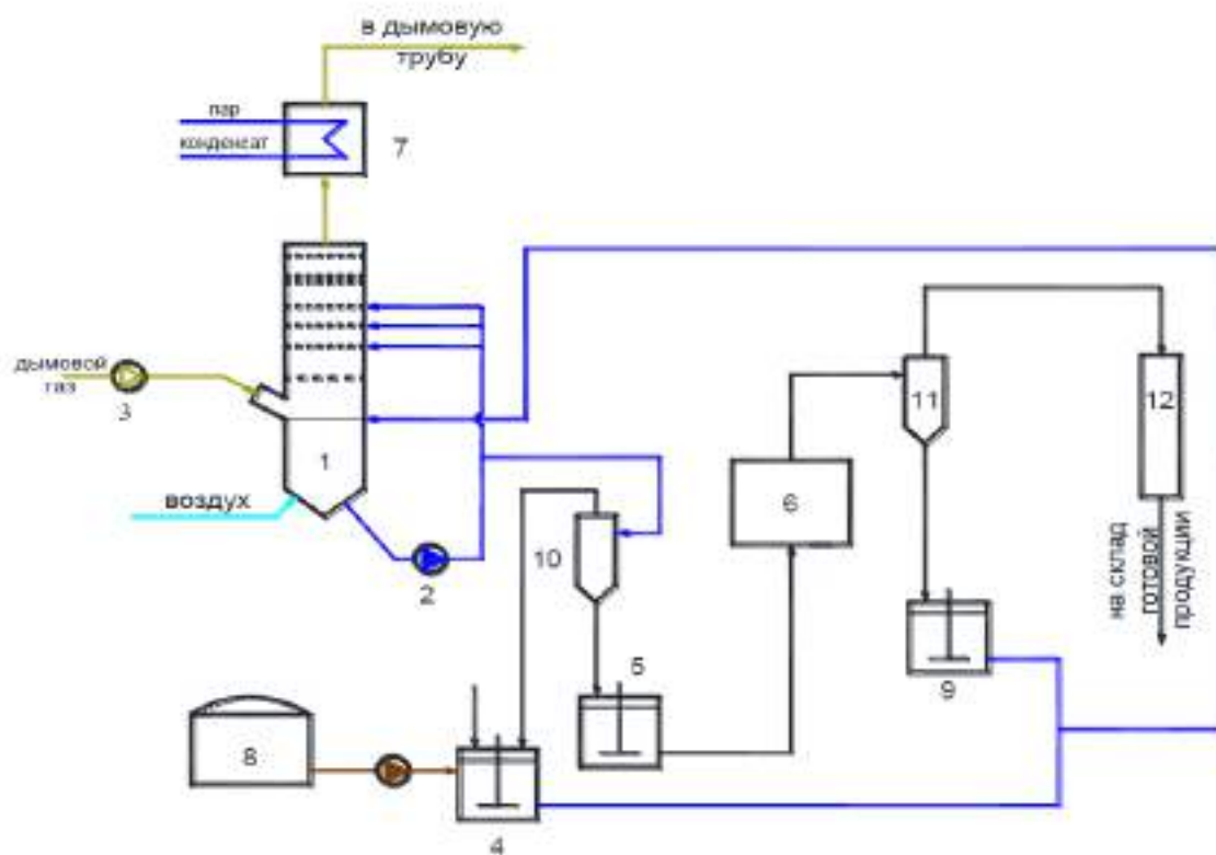
Рис.7.3 - Принципиальная технологическая схема установки аммиачно-сульфатной сероочистки
