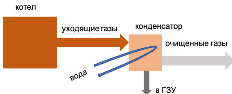
Рис.5.44 – Схема включение конденсатора дымовых газов
