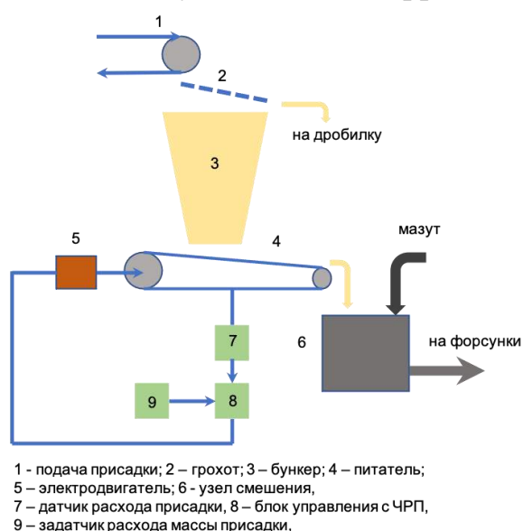
Рис.5.40 – Схема подачи присадки
