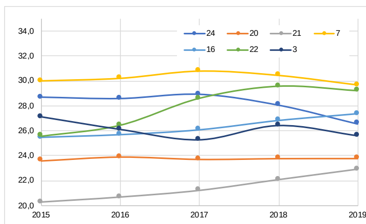
Рис.1.13 – КИТ ТЭЦ с КА на 8,8 МПа, %
