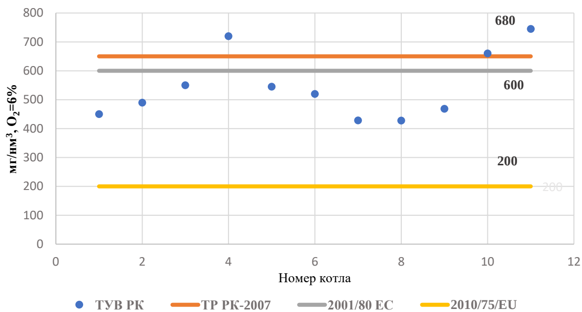
Рис. 5.25 – Удельные выбросы диоксида азота ( \text{NO}_x )
