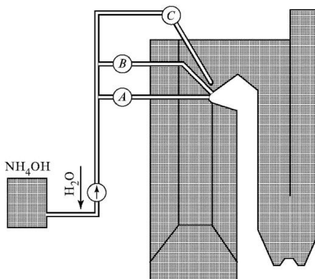
Рис. 4.29 - Различные способы ввода аммиачной воды в поток
