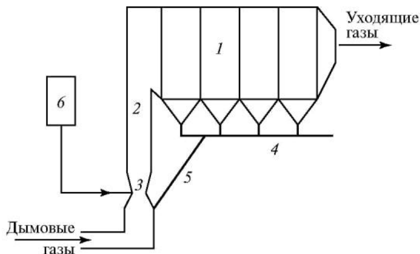
Рис.4.15 Схема установки сероочистки с циркулирующей инертной массой
