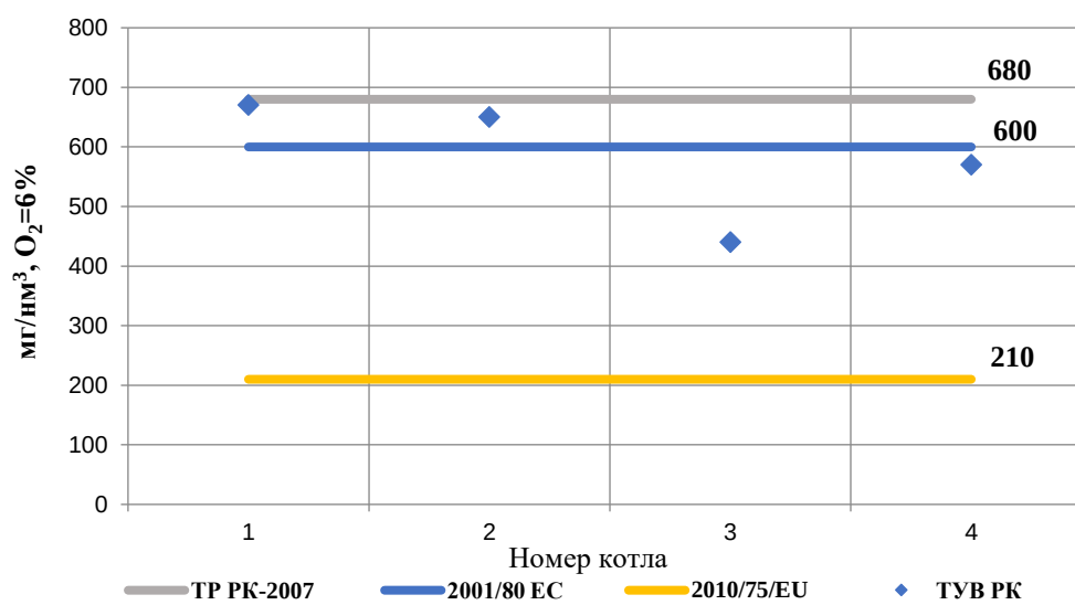
Рис.5.14 – Удельные выбросы диоксида азота ( \text{NO}_x )
