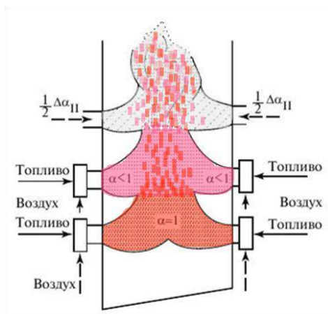
Рис.5.37 – Схема трехступенчатого сжигания
