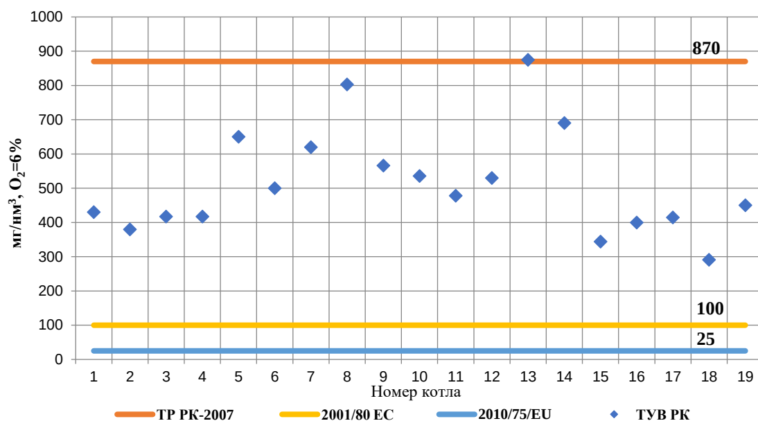
Рис. 5.17 – Удельные выбросы пыли за эмульгаторами при A_{пр} > 2,5 \text{ \% кг/МДж}
