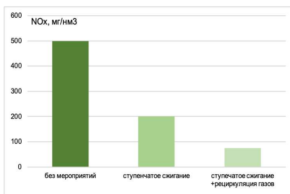
Рис.5.38 – Результаты комплексного применения методов подавления окислов азота на котлах ТГМ-96Б
