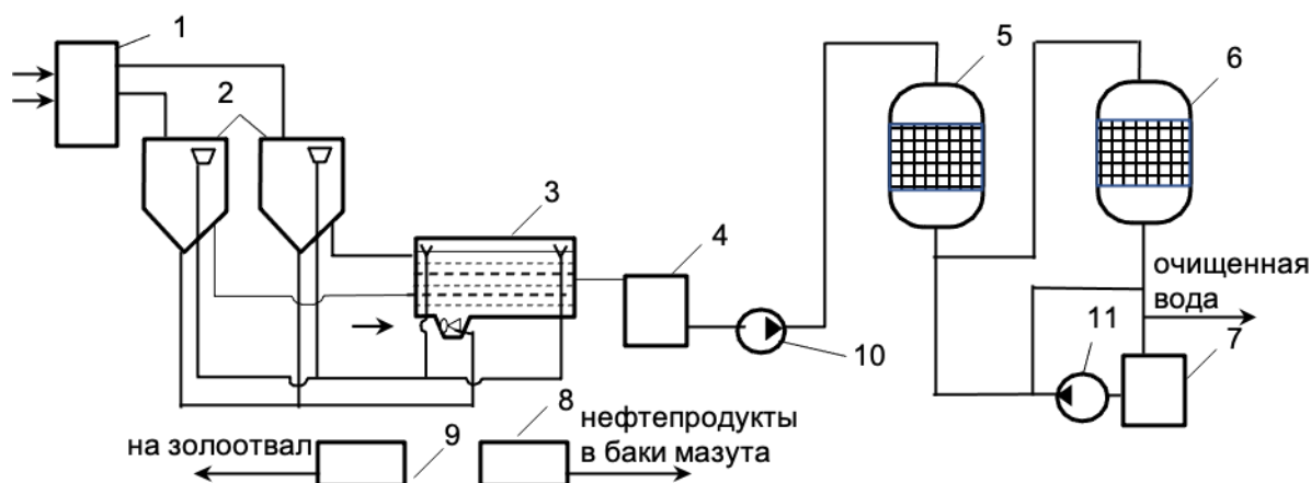
Рис. 4.41 - Схема установки очистки сточных вод, загрязненных нефтепродуктами
