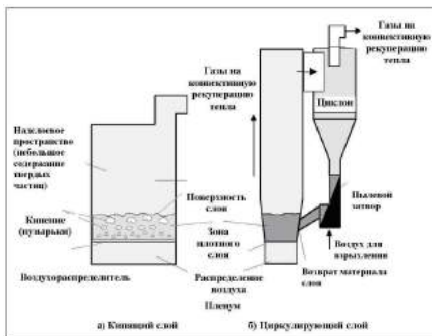
Рис.5.4 – Схемы сжигания угля в кипящем слое (ПКС и ЦКС)
