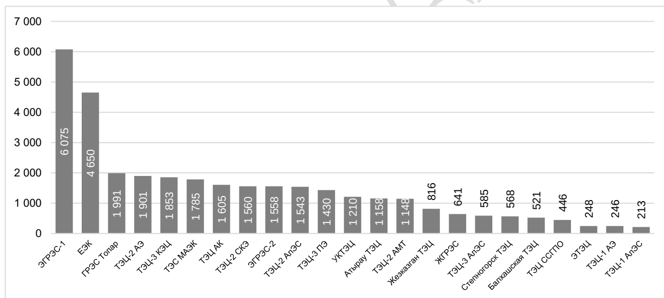
Рис. 1.15 - Расход условного топлива на ТЭС в 2019 году, тыс.т.ут (по данным КТА МЦЗТуИП)
