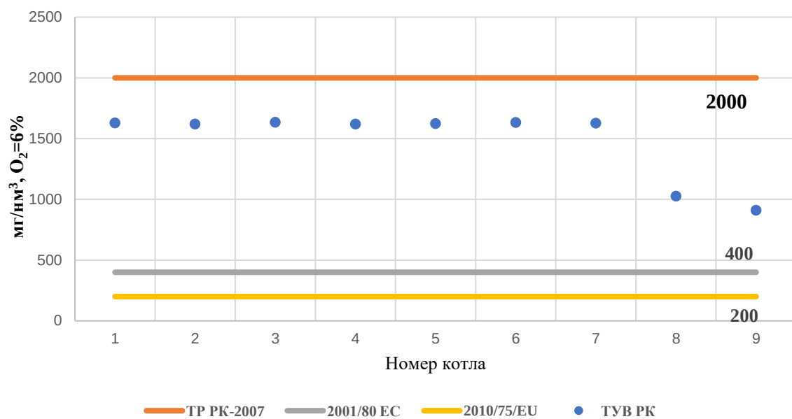
Рис. 5.30 – Удельные выбросы двуокиси серы (SO 2 )
