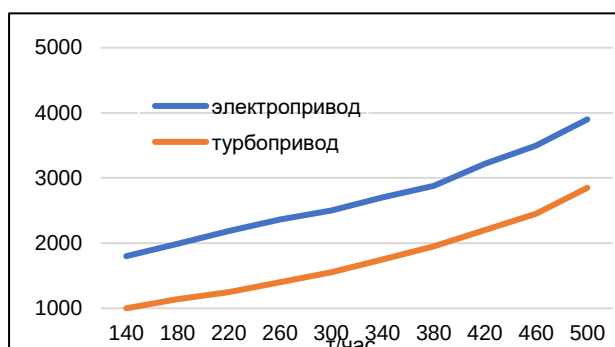
Рис.5.55 – Изменение мощности привода(кВт) от расхода питательной воды
