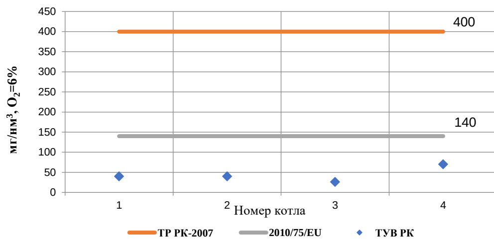
Рис.5.16 – Удельные выбросы окиси углерода ( \text{CO} )
