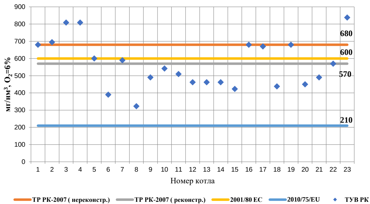
Рис. 5.19 – Удельные выбросы диоксида азота (NO x )
