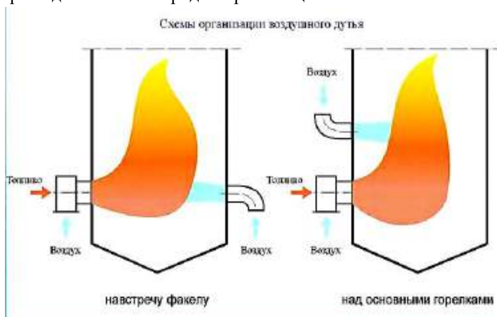
Рис. 4.22 - Схема технологии двухступенчатого сжигания
