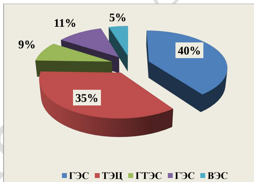
Рис.1.2 - Структура установленной мощности ТЭС РК по типу электростанций
