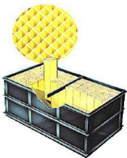
Рис. 4.32 - Сотовый катализатор
