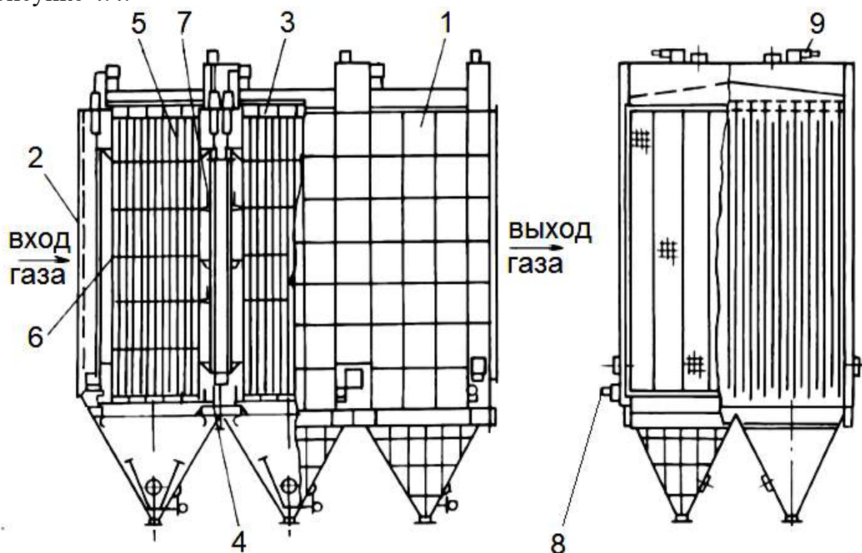
Рис. 4.4 - Трехпольный двухсекционный электрофилтр
