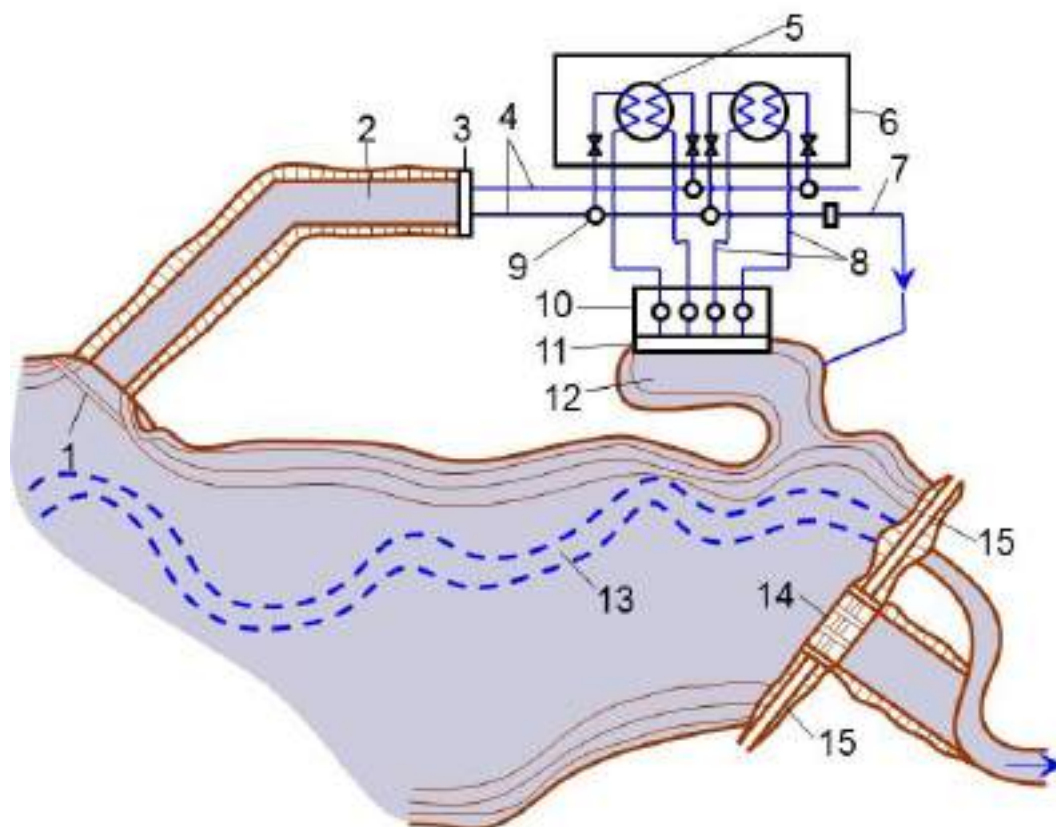
Рис. 3.22 - Обратная система технического водоснабжения ТЭС с водоемом -охладителем.
