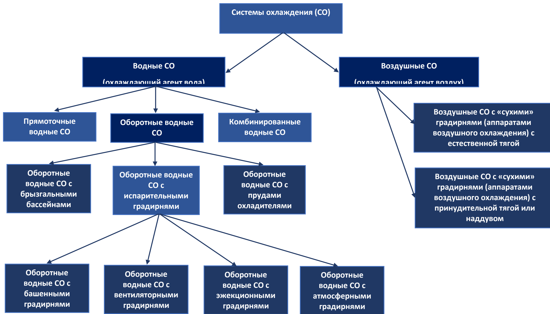
Рис. 3.23 - Классификация СО, применяемых в Казахстане
