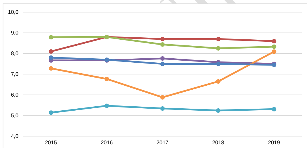
Рис.1.31 – Расход электроэнергии на СН по отпуску электроэнергии угольных КЭС СКД, блок 200 МВт на давление 140 кг/см 2 на газе, % (по данным КТА МЦЗТуИП)
