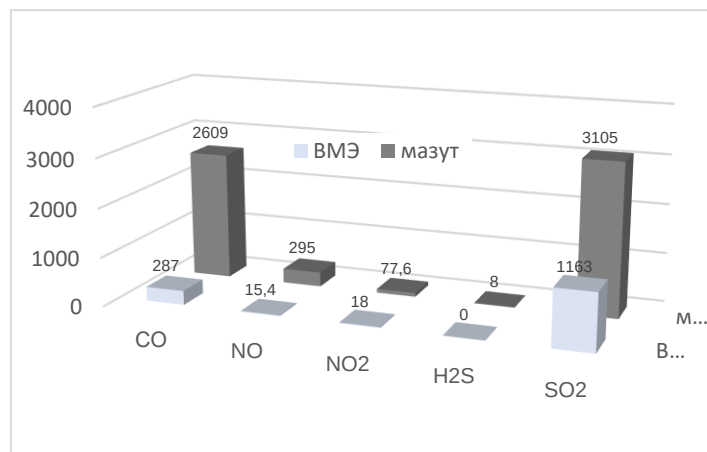
Рис.5.35 – Концентрации ЗВ при сжигании мазута и ВМЭ на котлах ТГМ-84
