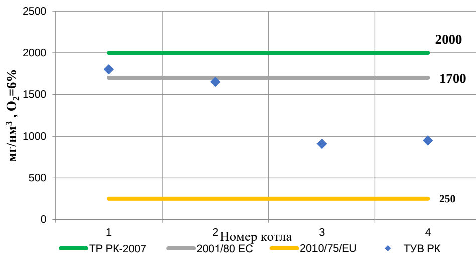
Рис.5.15 – Удельные выбросы двуокиси серы ( \text{SO}_2 )
