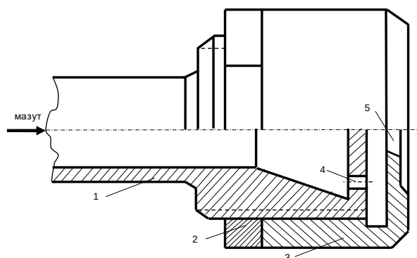
Рис.5.33 – Механическая форсунка
