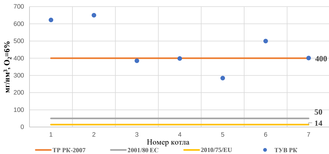
Рис.5.23 – Удельные выбросы пыли за эмульгаторами при A_{пр} > 2,5 % кг/МДж
