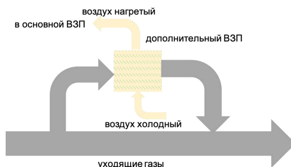
Рис. 4.46 – Схема установки дополнительного воздухоподогревателя на уходящих газах
