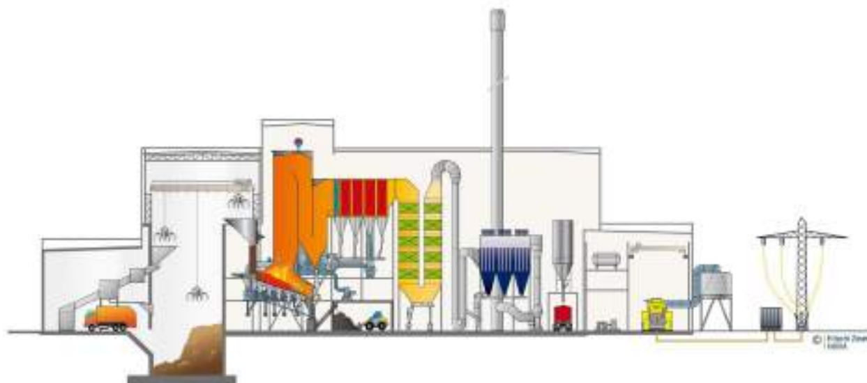
Рис. 5.48 - Схематическое представление предприятия термической переработки ТКО посредством прямого сжигания на движущейся решётке Edinburgh, UK Hitachi Zosen Inova
