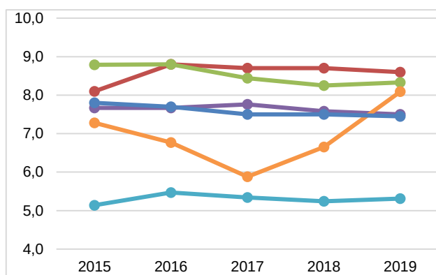
Рис. 1.23 - Расход ЭЭ на СН по отпуску электроэнергии ТЭЦ 13 МПа, % (по данным КТА МЦЗТуИП)
