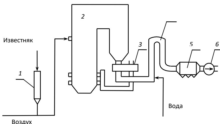
Рис. 4.14 - Схема сухой аддитивной очистки дымовых газов ТЭС от диоксида серы по технологии «Лифак»:
