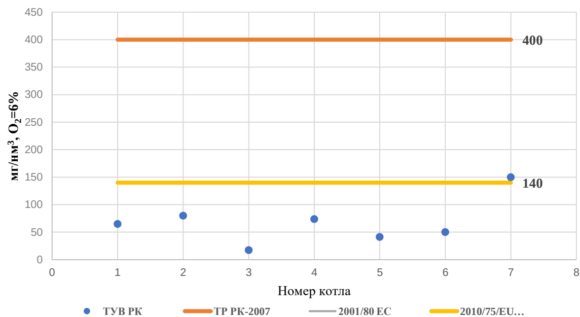
Рис. 5.27 – Удельные выбросы окиси углерода (CO)
