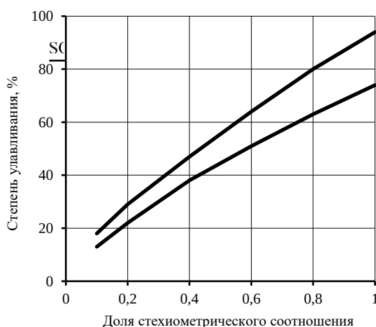
Рис. 4.34 - Зависимость степени улавливания SO_2 и NO_x от доли стехиометрического соотношения соответственно NH_3 и O_3
