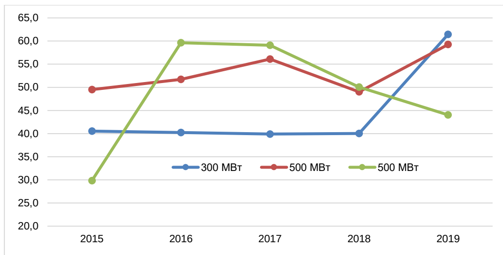
Рис.1.29 – Энергоемкость КЭС с угольными блоками 300 и 500 МВт, тут/млн.тенге, [17]
