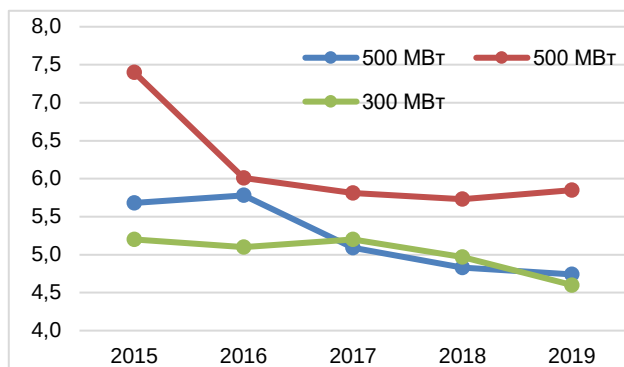
Рис. 1.21 – Расход ЭЭ на СН блоков 300 и 500 МВт (по данным КТА МЦЗТуИП)
