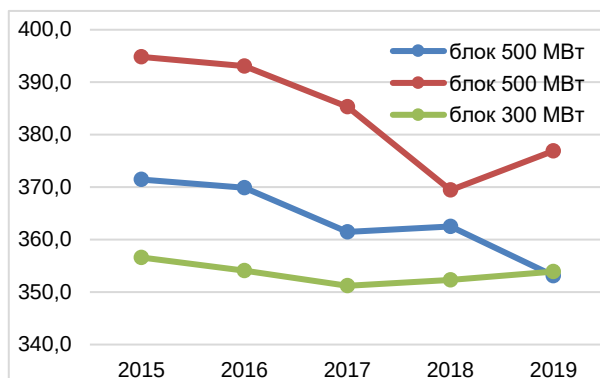
Рис. 1.16 – УРУТ по отпуску электрической энергии КЭС с пылеугольными блоками 500 и 300 МВт, г/кВтч (по данным КТА МЦЗТ и ИП)
