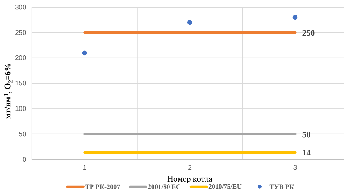
Рис. 5.24 – Удельные выбросы пыли за эмульгаторами при A_{\text{пр}} \leq 2,5 \text{ \% кг/МДж}
