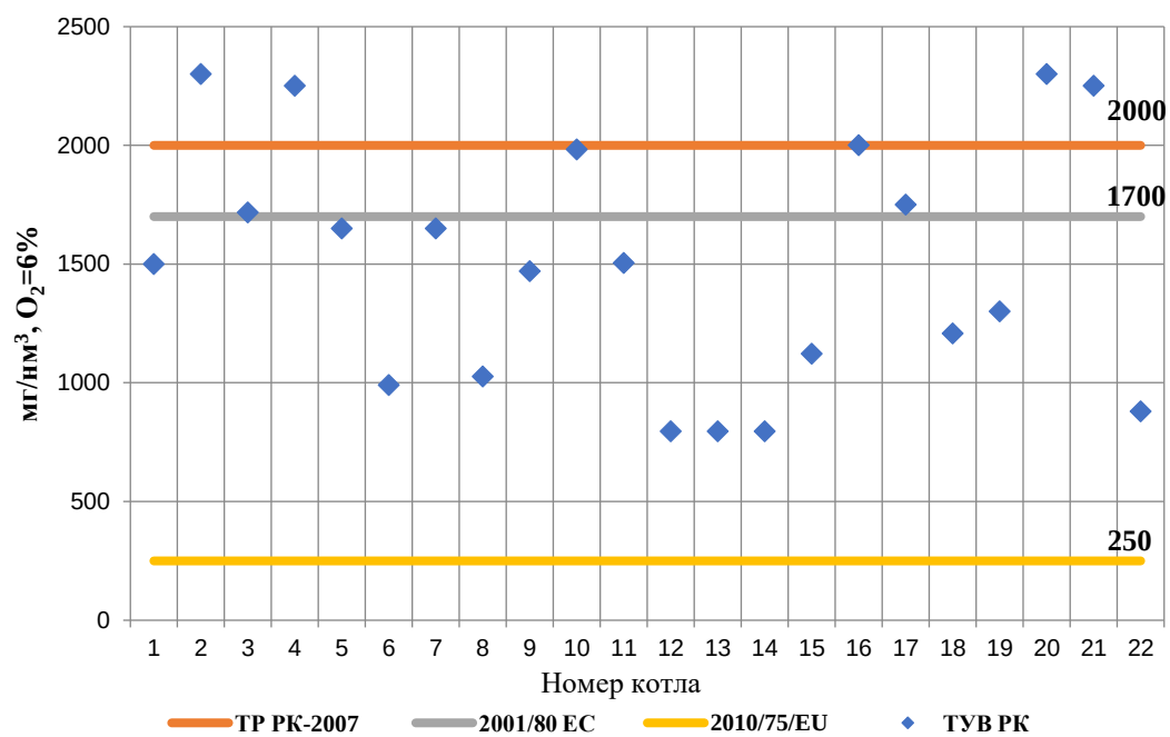
Рис. 5.20 – Удельные выбросы двуокиси серы (SO 2 )
