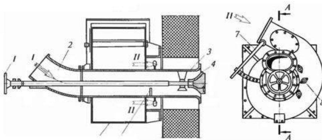
Рис. 5.2 - Вихревая пылеугольная горелка ОРГРЭС
