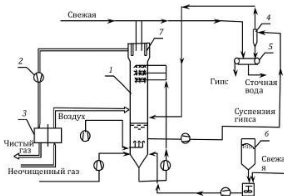
Рис. 4.10 - Принципиальная схема установки сероулавливания по технологии фирмы «Бишофф»:
