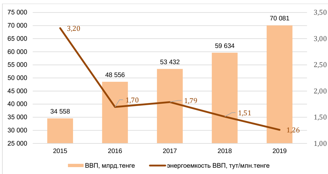
Рис.1.27 - Динамика ВВП и энергоёмкости ВВП РК за 2015-2019 годы, [17]
