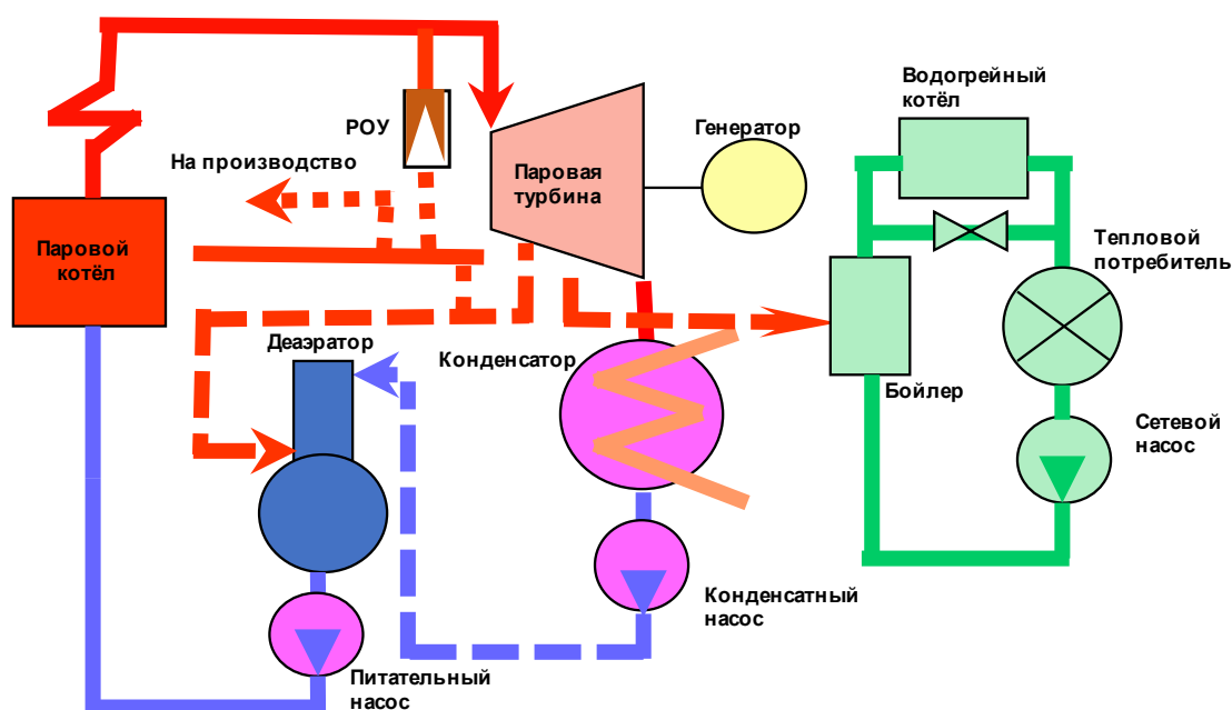
Рис.3.3 – Принципиальная тепловая схема ТЭЦ
