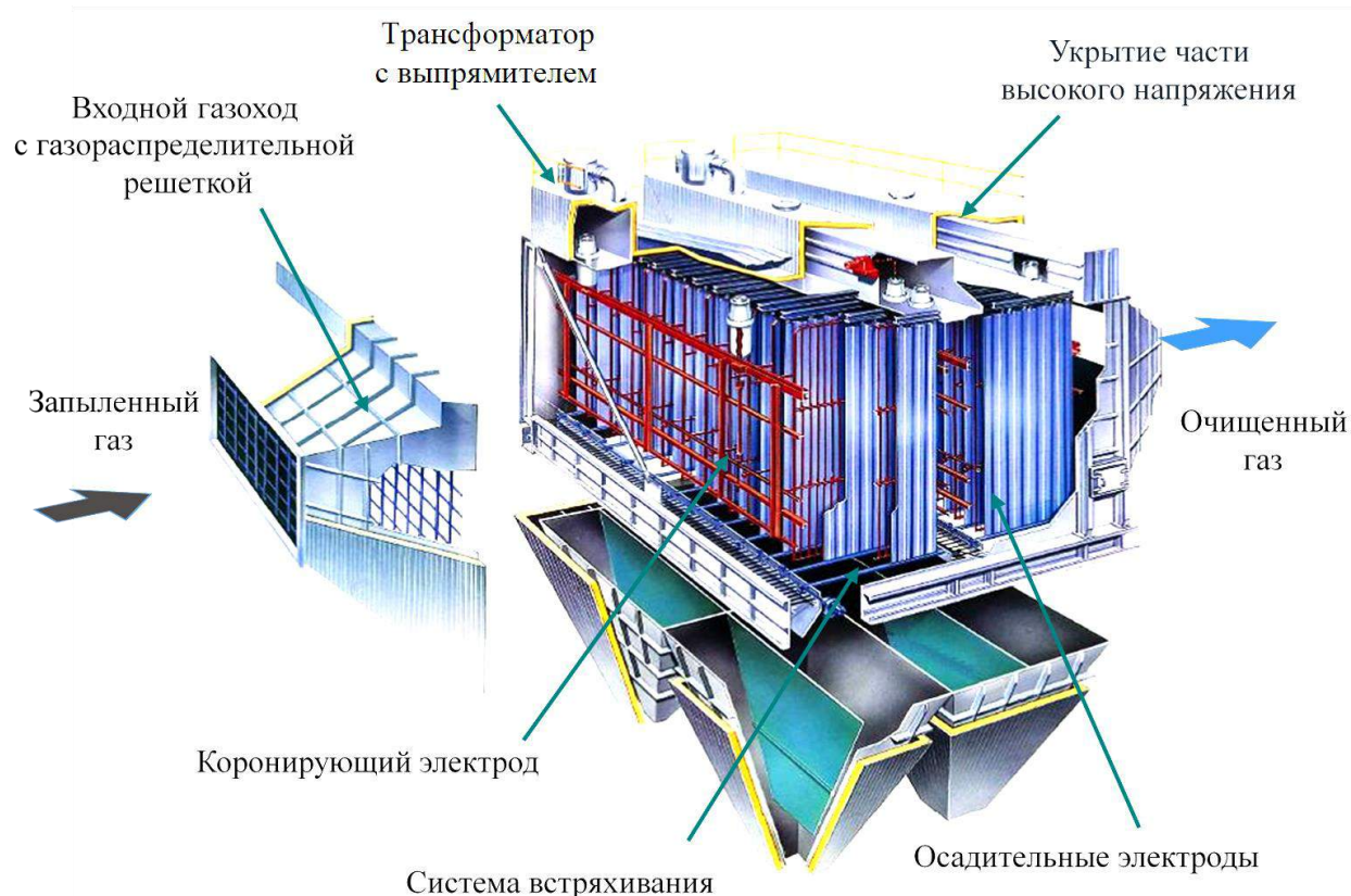
Рис. 4.3 - Общий вид стандартного сухого электрофильтра
