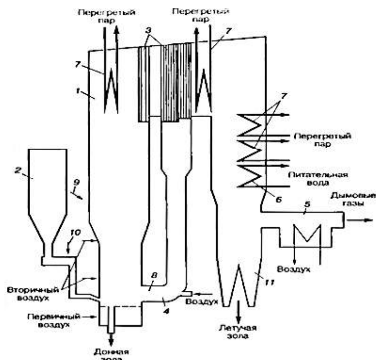
Рис. 5.11 - Принципиальная схема котла ЦКС «Бабкок-Вилькокс»
