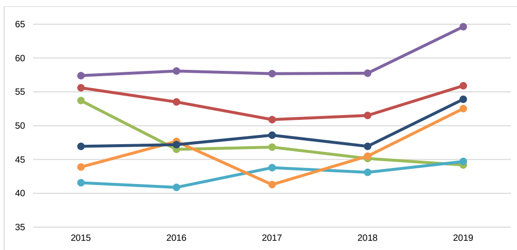
Рис.1.33 – Расход электроэнергии на СН по отпуску тепловой энергии угольных ТЭЦ 140 кг/см 2 , кВтч/Гкал (по данным КТА МЦЗТиИП)
