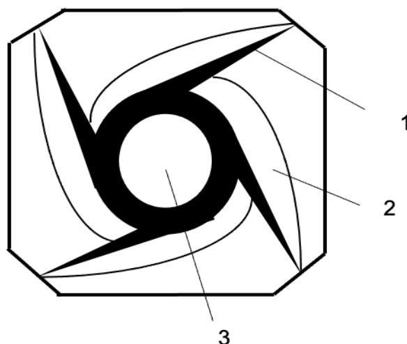
Рис. 4.24 – Принципиальная схема концентрического сжигания:
