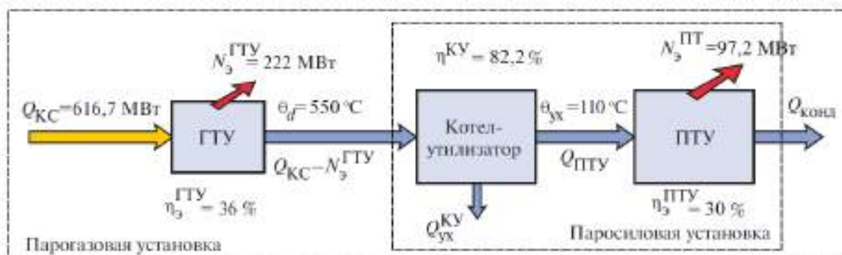
Рис. 3.13 - Диаграмма потоков мощности в утилизационной ПГУ
