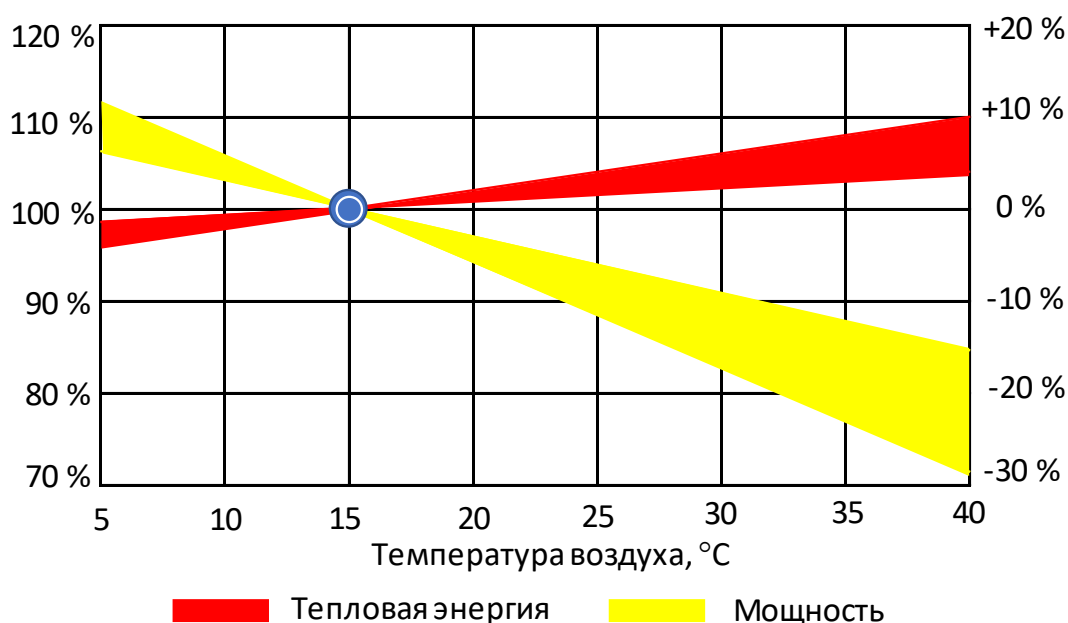
Рис. 7.4 - Производительность ГТУ в зависимости от температуры окружающего воздуха
