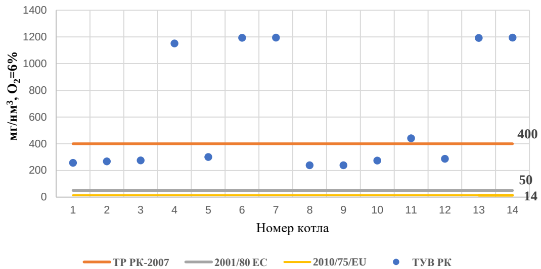
Рис. 5.22 – Удельные выбросы пыли за электрофильтрами при A_{пр} > 2,5 % кг/МДж
