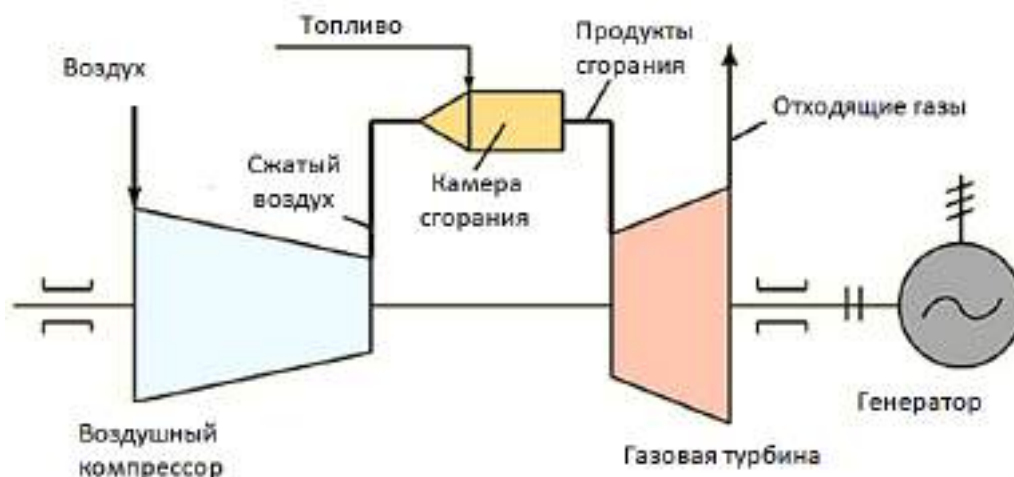
Рис. 3.5 - Принципиальная схема простейшей ГТУ
