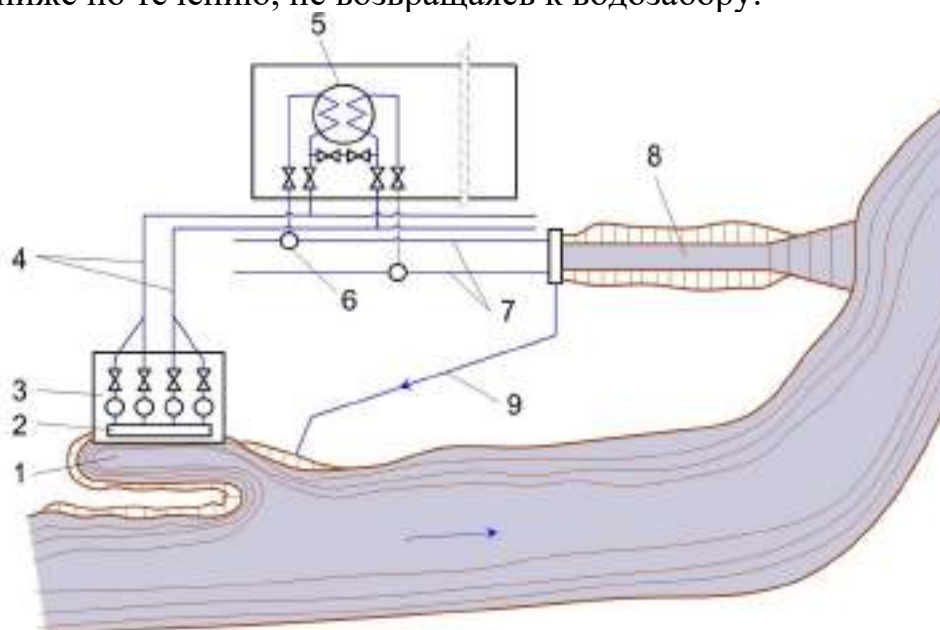
Рис. 3.21 - Прямоточная система технического водоснабжения ТЭС
