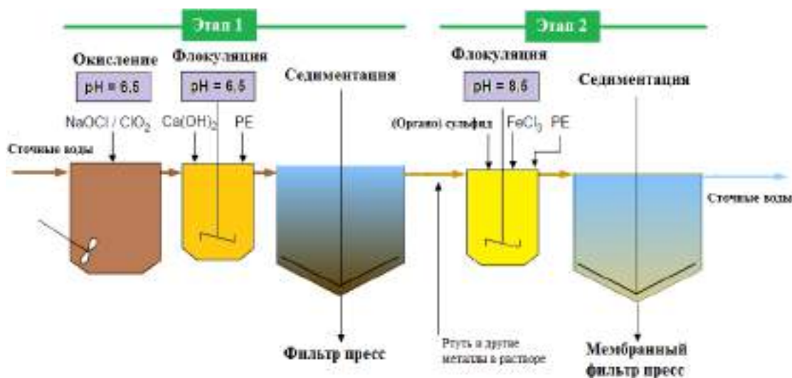
Рис. 4.44 - Станция двухэтапной очистки сточных вод
