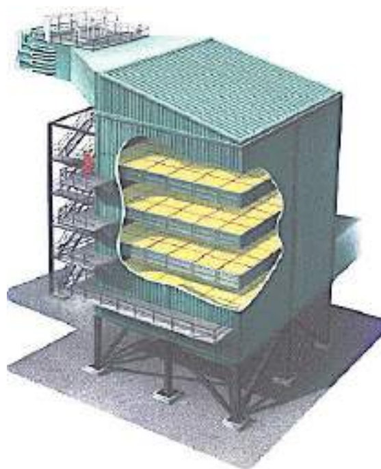
Рис. 4.33 - Пример реактор с четырьмя слоями катализатора
