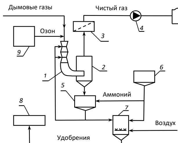
Рис. 4.35 – Принципиальная технологическая схема установки одновременной очистки дымовых газов от оксидов серы и азота: 1 – скруббер; 2 – каплеуловитель; 3 – подогреватель; 4 – дымосос; 5 – циркуляционная емкость; 6 – емкость аммонийного раствора; 7 – реактор; 8 – узел подготовки удобрений; 9 – озонатор
