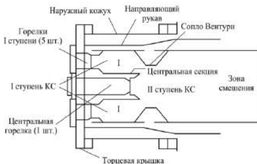
Рис. 3.8 - Принципиальная схема КС типа DLN фирмы GE
