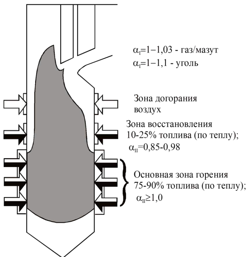
Рис. 4.23 - Схема организации трехступенчатого сжигания
