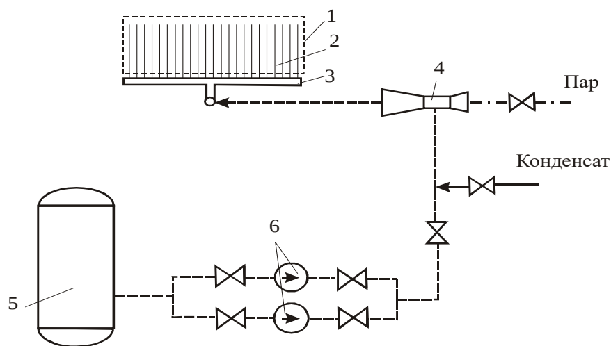
Рис. 4.30 - Принципиальная технологическая схема (СНКВ) установки на Тольяттинской ТЭЦ
