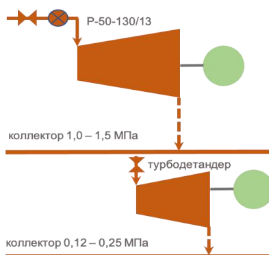
Рис.5.58 – Схема включения турбодетандера
