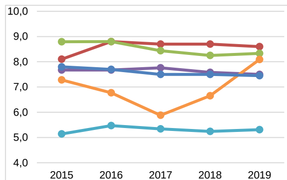
Рис.1.22 – Расход ЭЭ на СН по отпуску ЭЭ ТЭЦ 13 МПа (по данным КТА МЦЗТуИП)
