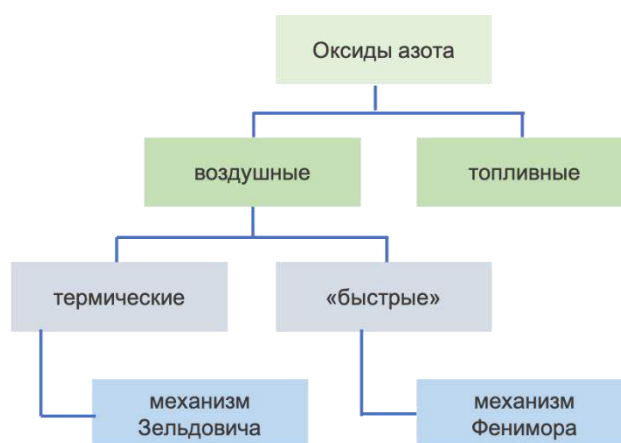
Рис. 4.17 - Схема источников образования оксидов азота
