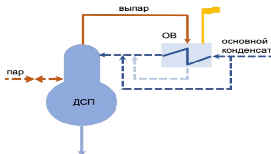
Рис.5.64 – Схема включения охладителя выпара
