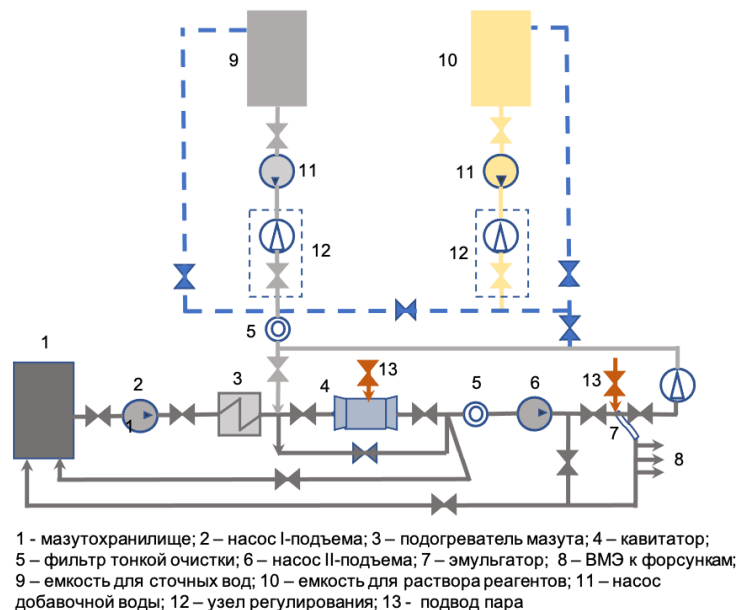
Рис.5.39 – Комбинированная схема подготовки ВМЭ
