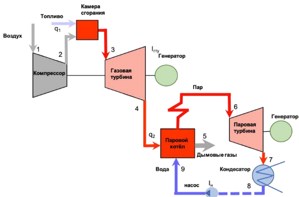
Рис.3.4 – Схема ПГУ
