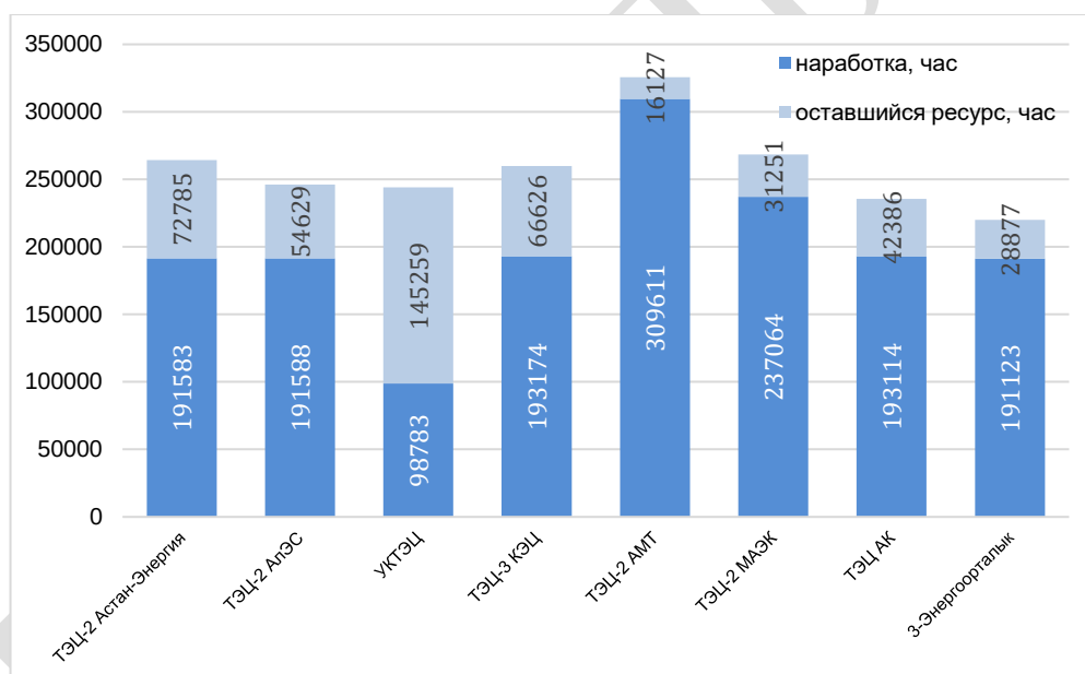
Рис. 1.6 - Средняя наработка турбоагрегатов давлением пара 130 кг/см 2
