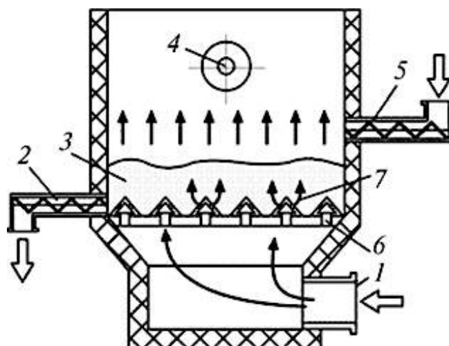
Рис. 5.49 - Топка со стационарным (пузырьковым) кипящим слоем
