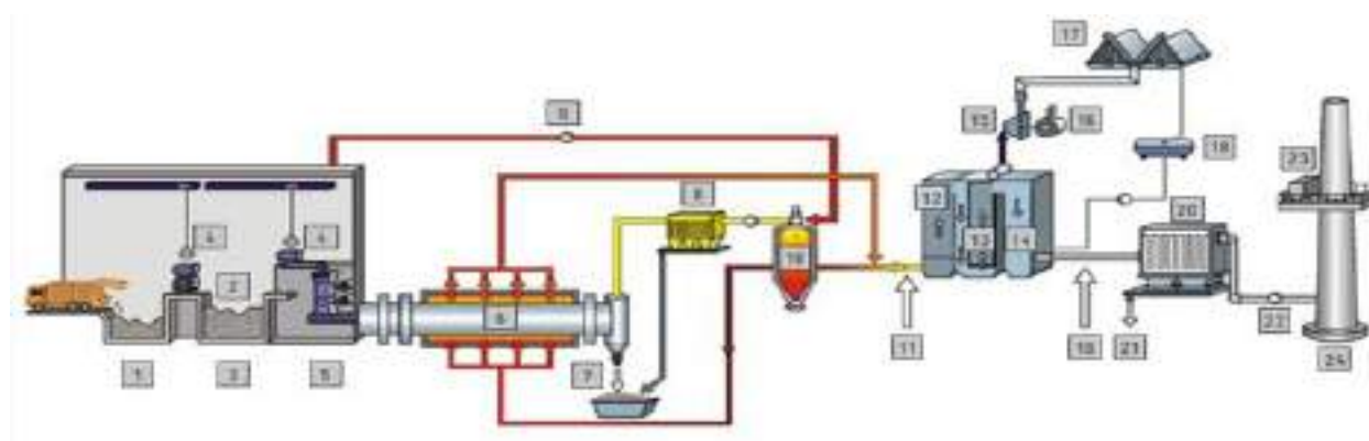
Рис. 5.53- Схема предприятия по термической переработке ТКО в энергию с помощью пиролиза
