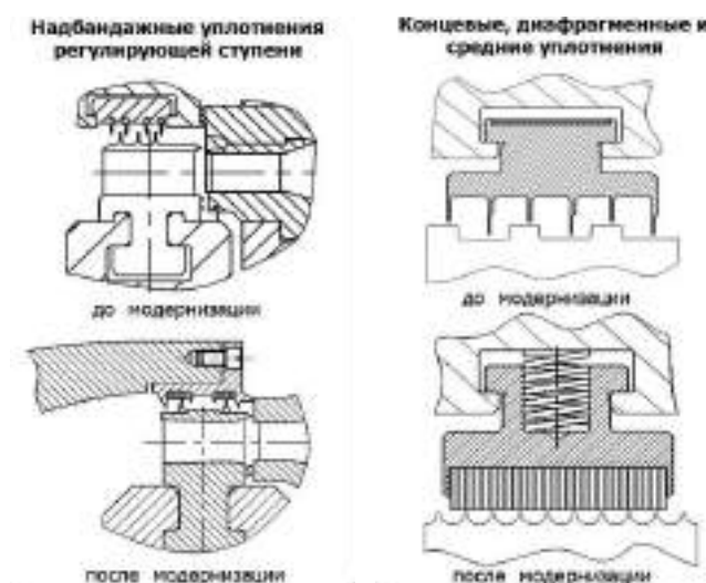
Рис.5.61 – Схема установки сотовых уплотнений
