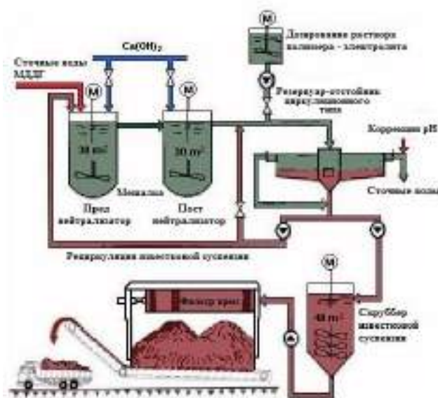
Рис. 4.43 - Установка очистки сточных вод мокрой системы десульфуризации
