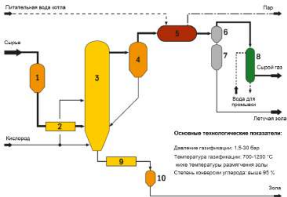
Рис. 3.15 - Технологическая схема высокотемпературной газификации по Винклеру 1-Загрузочный бункер; 2-Загрузочный шнек; 3-Газогенератор высокотемпературный по Винклеру; 4-Циклонный сепаратор; 5-Котел-утилизатор; 6-Фильтр; 7-Воронка-затвор; 8-Мокрая очистка от пыли; 9-Охлаждающий шнек; 10- Система воронок-затворов;
