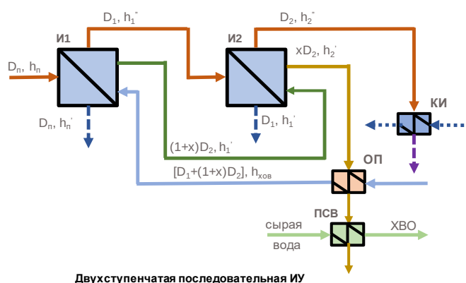
Рис.5.56 - Схема двухступенчатой последовательной испарительной установки
