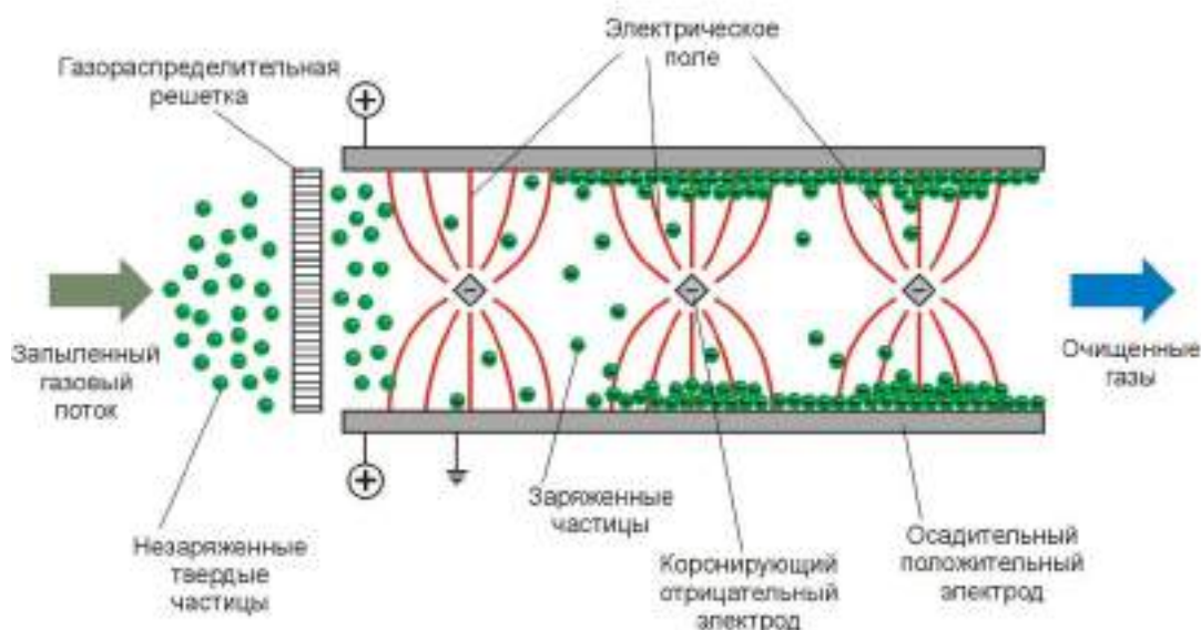
Рис. 4.2 - Принцип работы электрофильтра
