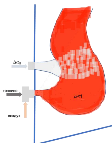
Рис.5.36 – Схема двухступенчатого сжигания
