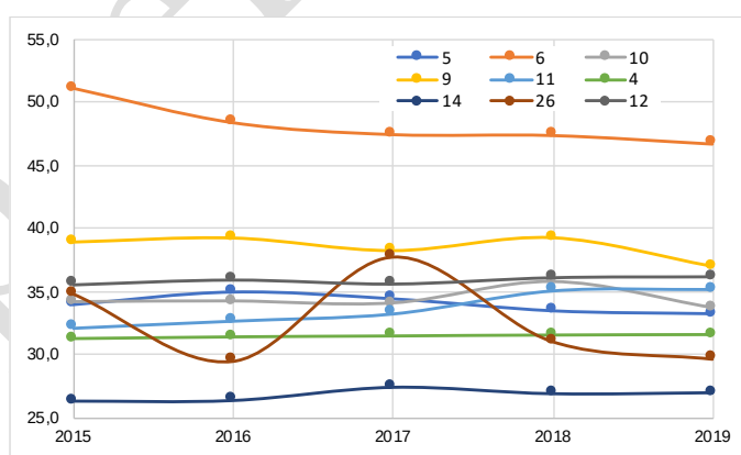
Рис.1.12 – КИТ ТЭЦ с КА на 13,8 МПа, % 5, 6, 10, 9, 11, 4 – БКЗ-420-140; 12 – БКЗ-320-140; 14 – ТГМ-96Б; 26 – ТГМЕ-464
