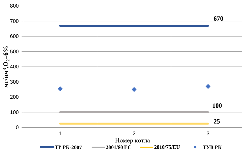
Рис.5.13 – Удельные выбросы пыли за эмульгаторами при A_{пр} \leq 2,5 \% \cdot \text{кг/МДж}
