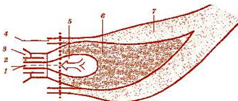
Рис. 4.20 - Факел малотоксичной горелки со ступенчатой подачей воздуха:
