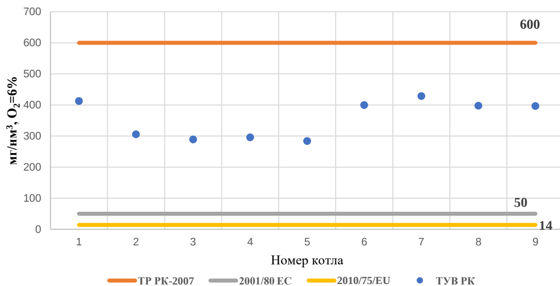
Рис.5.28 – Удельные выбросы пыли
