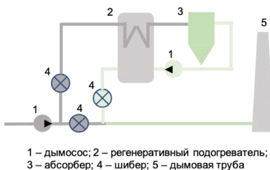
Рис.5.42 – Мокрая известковая схема очистки от окислов серы
