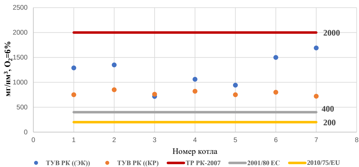
Рис. 5.26 – Удельные выбросы двуокиси серы (SO 2 )
