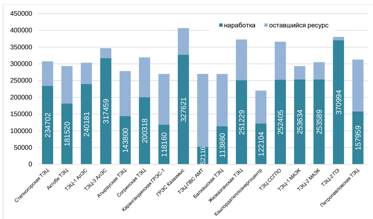
Рис. 1.7 - Средняя наработка турбоагрегатов на давление пара 90 кг/см 2
