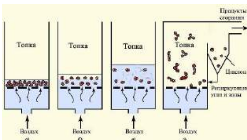
Рис.5.1 - Основные технологические схемы сжигания угля в топочной технике
