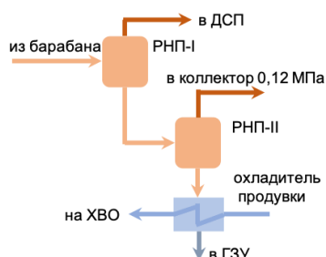
Рис.5.65 – Схема двухступенчатого РНП
