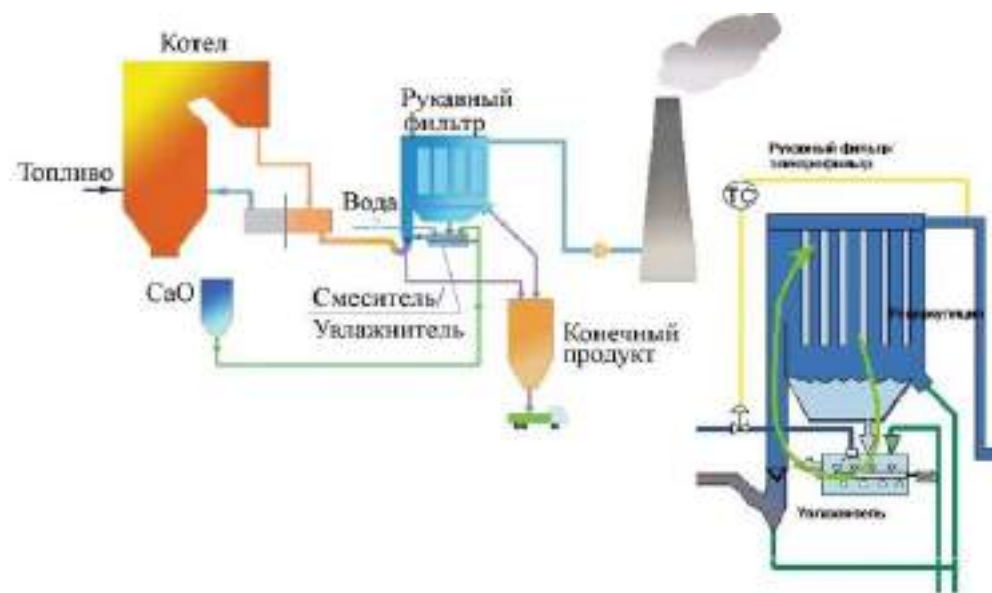
Рис. 4.16 - Схема полусухой сероочистки по NID технологии Alstom
