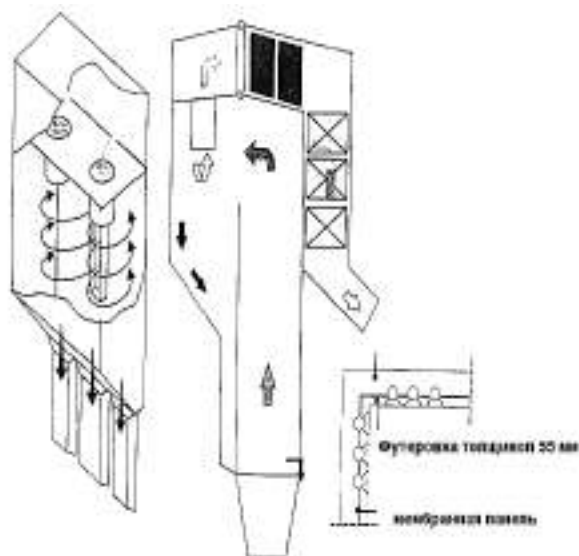
Рис. 5.8 - Схема компактных сепараторов золы
