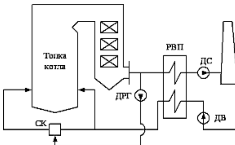
Рис. 4.26 - Типичная схема рециркуляции дымовых газов в топку котла
