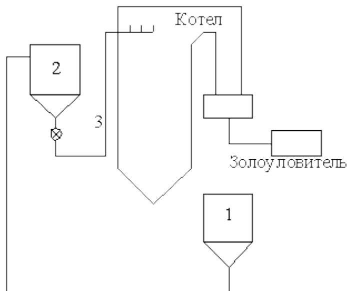
Рис. 4.9 - Принципиальная схема сероочистки по СИТ (сухой известняковой очистки)
