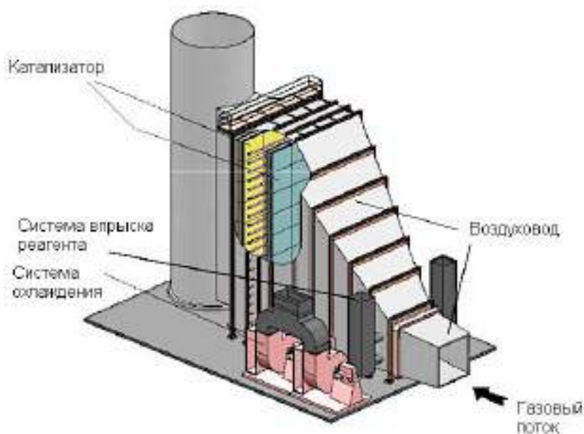
Рис. 4.31 - Система СКВ
