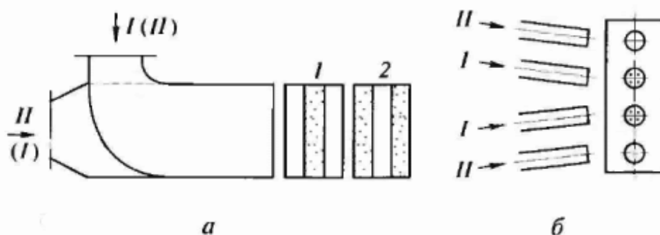
Рис. 5.3 - Принципиальная схема прямоточных горелок
