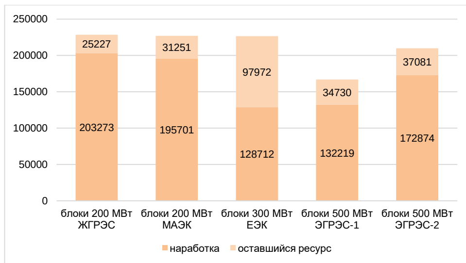
Рис.1.5 - Средняя наработка генерирующего оборудования блочных ТЭС
