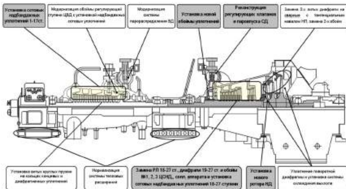
Рис.5.56 – Схема реконструкции ПТ-80-130/13
