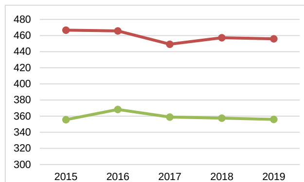
Рис. 1.17 – УРУТ по отпуску электрической энергии КЭС с газомазутными блоками 200 МВт, г/кВтч (по данным КТА МЦЗТ и ИП)
