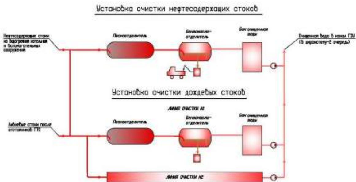
Рис. 4.42 - Схема установки очистки нефтесодержащих стоков совместно с очисткой поверхностного стока с территории
