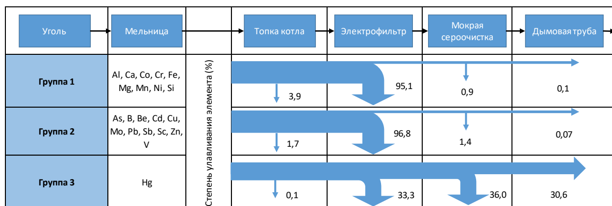
Рис. 4.38 - Массовый баланс тяжелых металлов на электростанциях, работающих на угле
