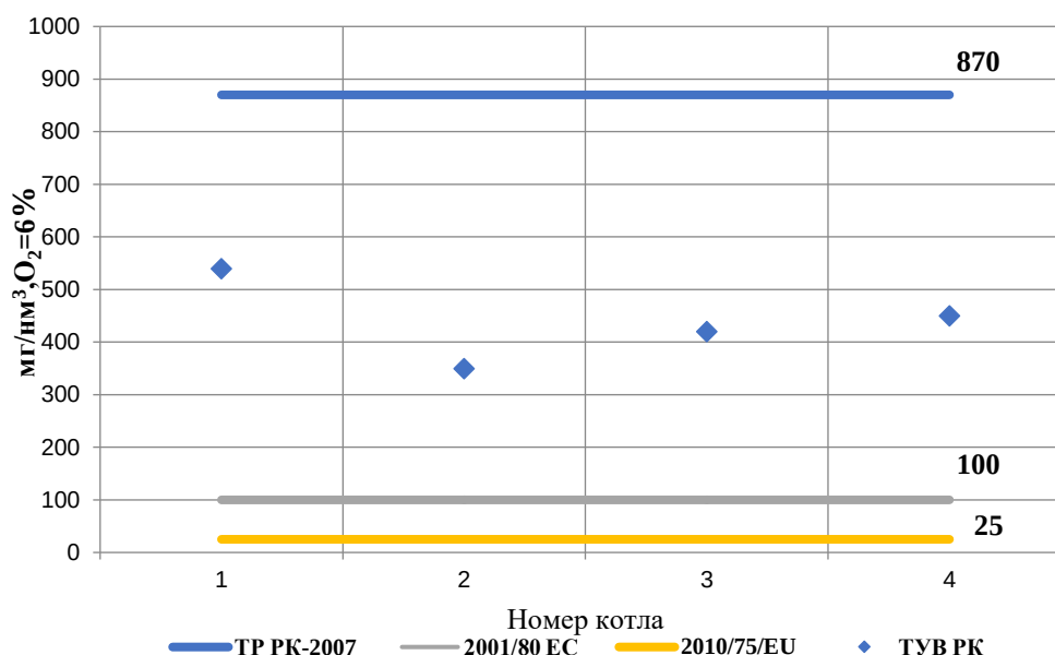
Рис.5.12 – Удельные выбросы пыли за эмульгаторами при A_{пр} > 2,5 \text{ \% кг/МДж}
