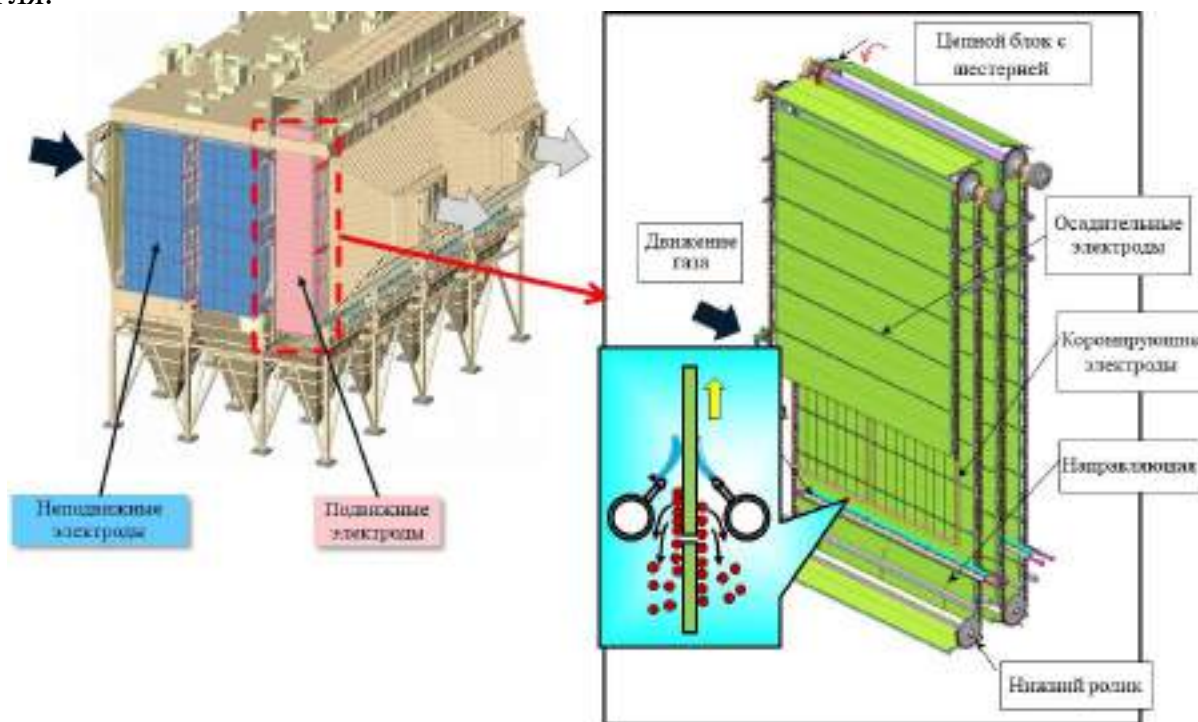
Рис.4.5 - Электрофильтр с подвижными электродами
