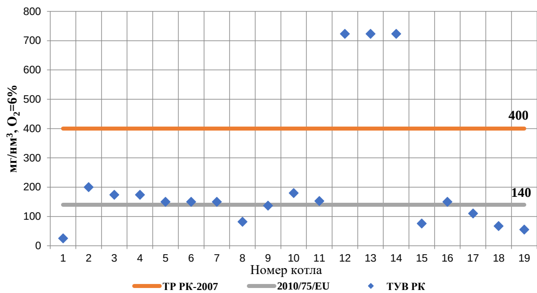
Рис. 5.21 – Удельные выбросы окиси углерода (CO)
