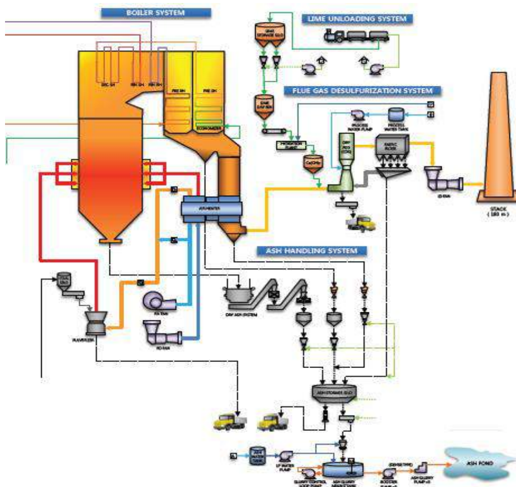
Рис. 5.31 - Блок-схема комбинированной системы ЗШУ с отгрузкой потребителям сухой золы из УОСЗ и шлака из-под котлов
