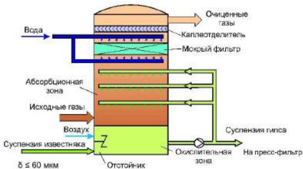
Рис. 4.12 - Конструкция абсорбера мокрой сероочистки [37]
