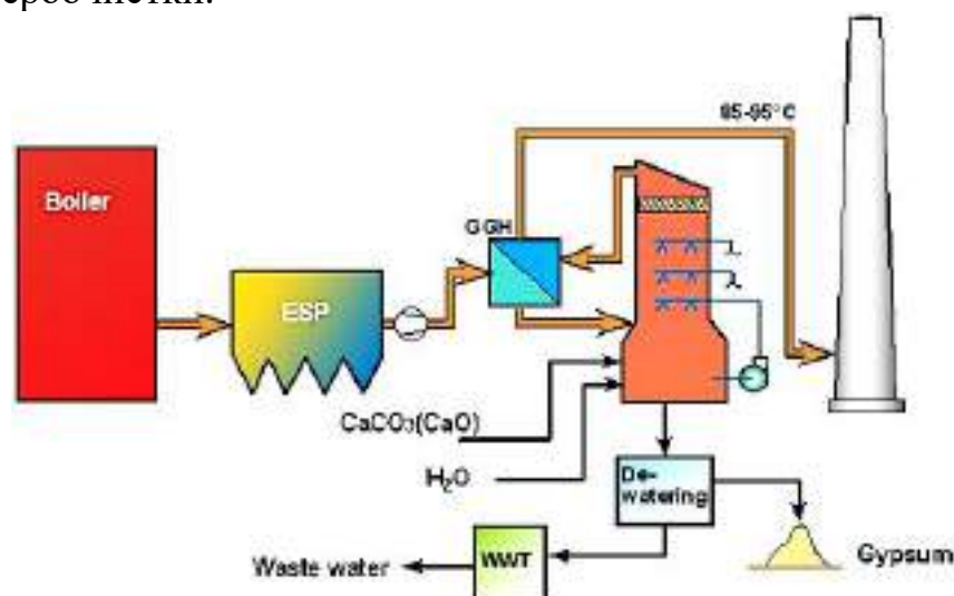
Рис. 4.11 - Типичная технологическая линия мокрой сероочистки [37]
