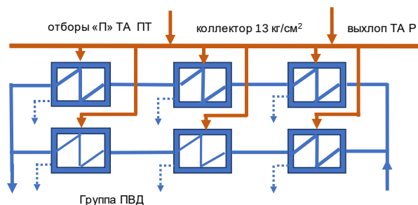
Рис.5.55 - Групповая схема включения ПВД
