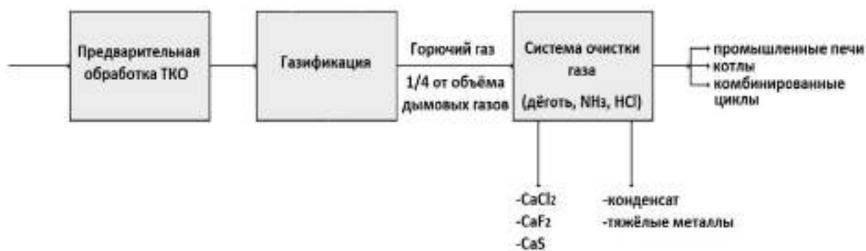
Рис. 5.51 - Блок-схема обычного процесса газификации ТКО
