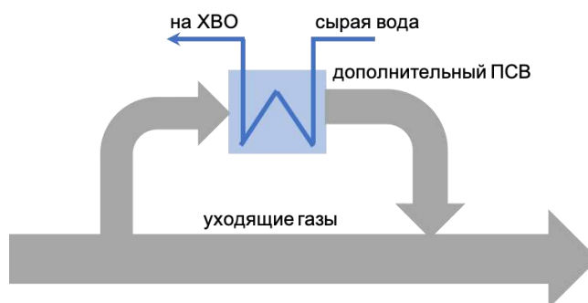
Рис.4.47 – Схема включения дополнительного ПСВ от уходящих газов
