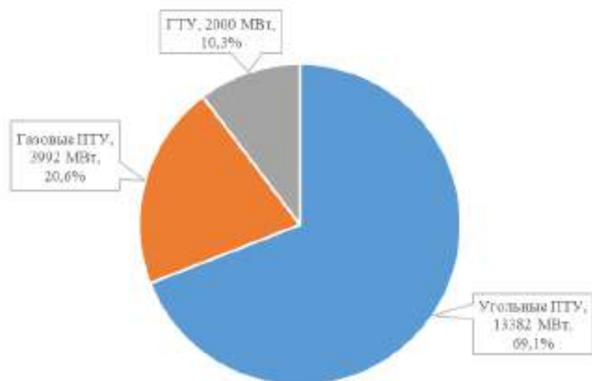
Рис. 1.10 - Структура ТЭС Казахстана по технологии производства энергии
