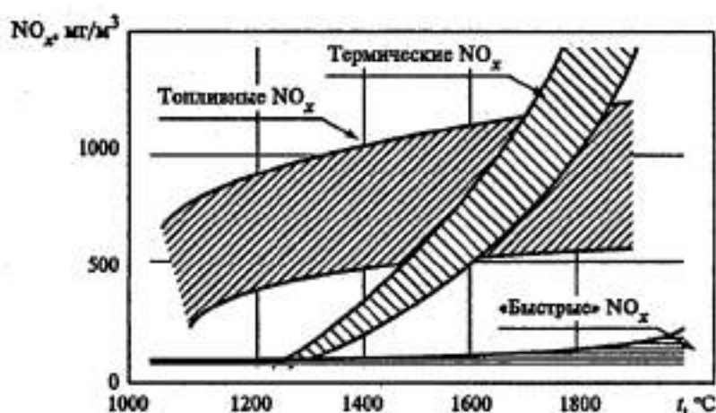
Рис.4.18 - Зависимость образования оксидов азота от температуры при сжигании органического топлива
