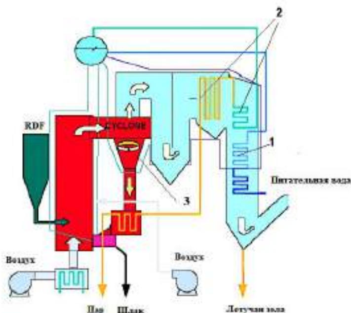
Рис.5.50 - Котел с ЦКС для сжигания бытовых отходов, установленный на предприятии Lomellina (Италия) [24]
