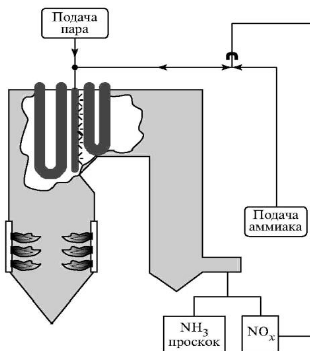
Рис. 4.28 - Схема организации процессов СНКВ
