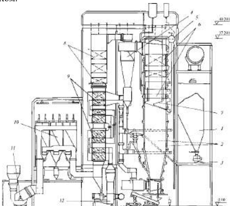
Рис. 5.10 - Котел с ЦКС по схеме «Циркофлюид»:
