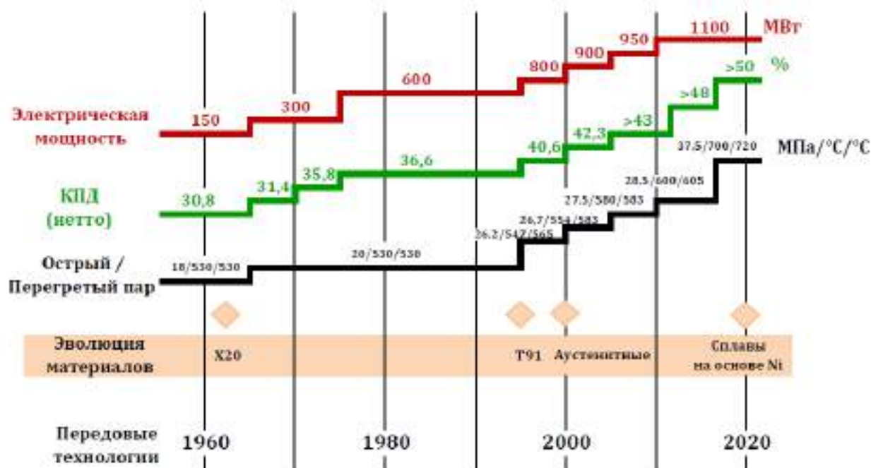
Рис. 7.1 - Тренд повышения начальных параметров пара на ТЭС в Японии
