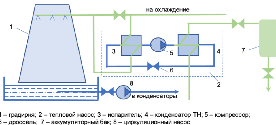
Рис.5.63 – Схема работы теплового насоса, включенного с градирней
