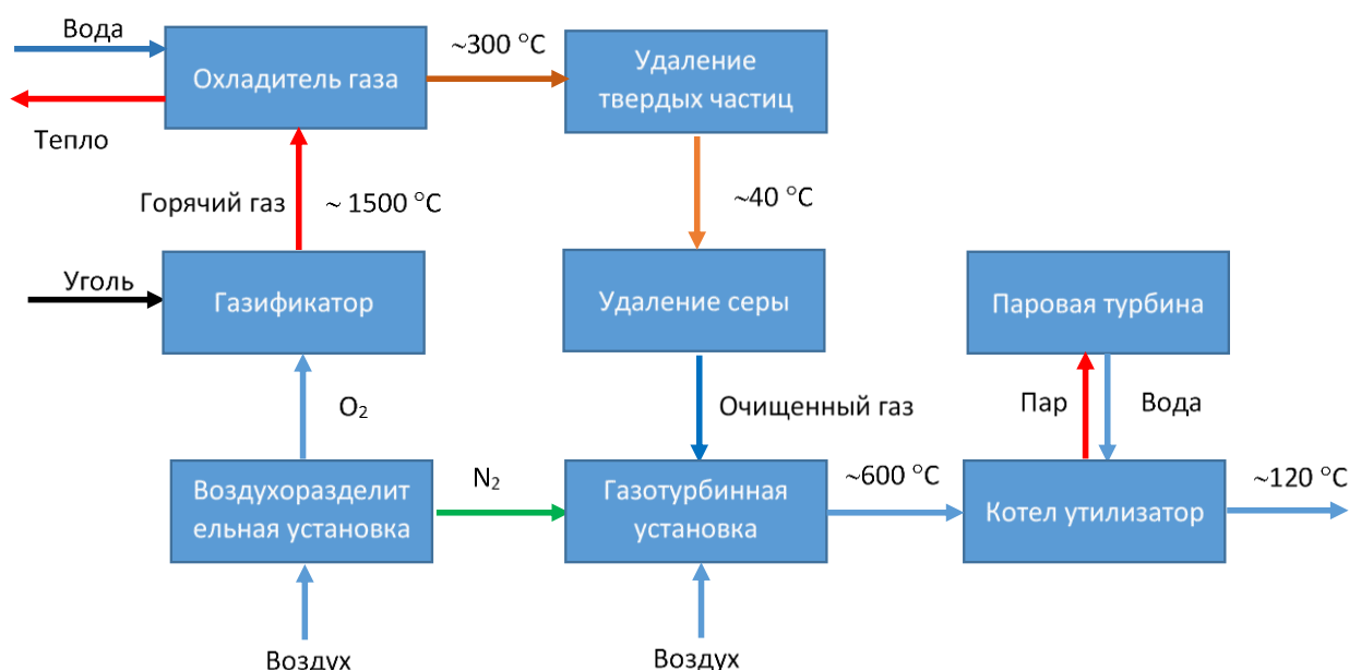
Рис. 3.17 - Блок-схема процессов в цикле ПГУ с ВЦГ
