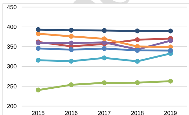
Рис 1.18 – УРУТ по отпуску электроэнергии угольных ТЭЦ с КА типа Е-420-140 (по данным КТА МЦЗТ и ИП)
