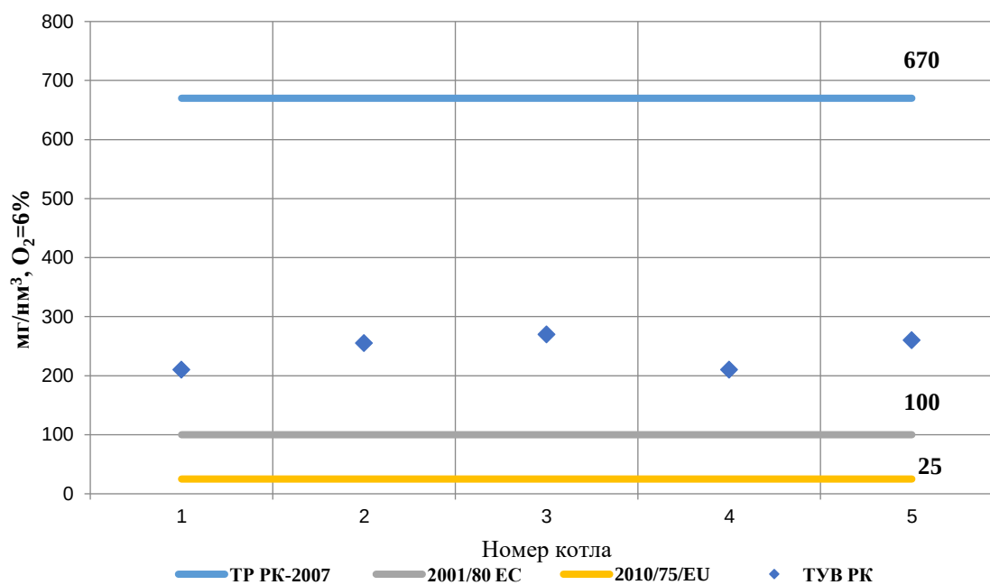
Рис. 5.18 – Удельные выбросы пыли за эмульгаторами при A_{пр} \leq 2,5 \text{ \% кг/МДж}
