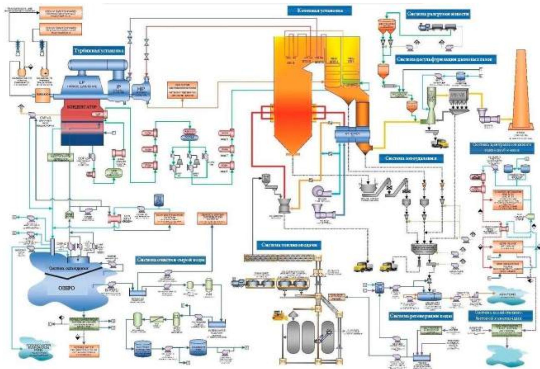
Рис. 1.34 - Общая схема топливосжигающей установки
