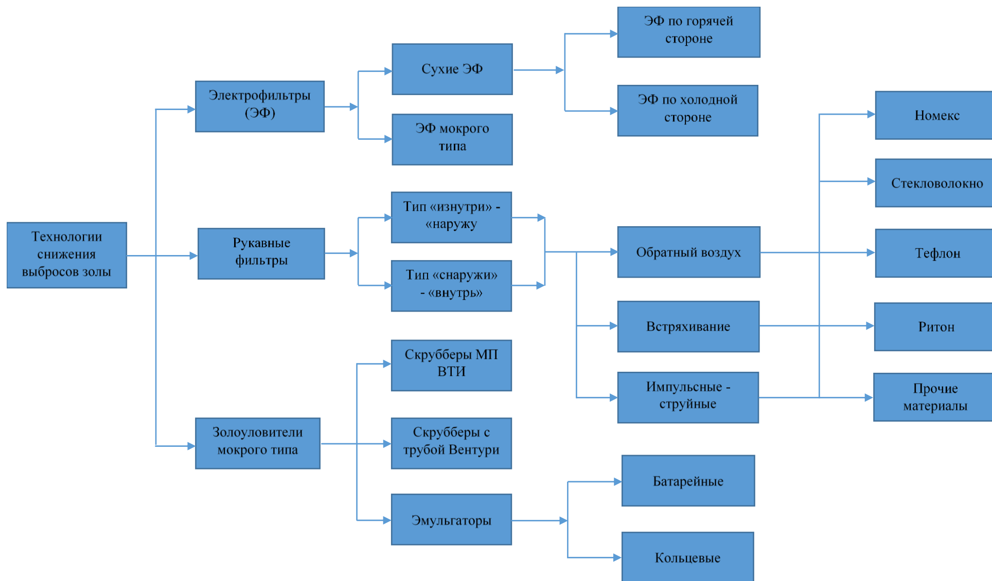
Рис. 4.1 - Обзор золоулавливающих установок
