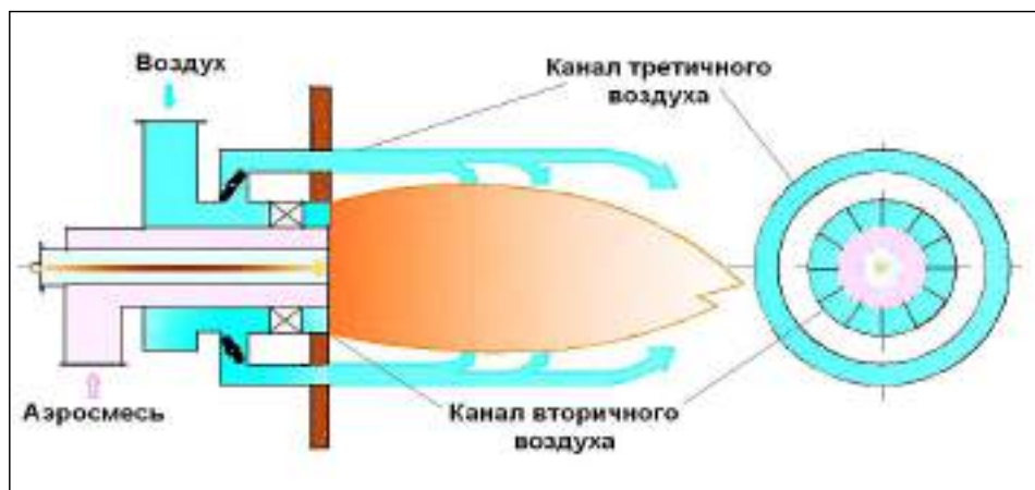
Рис. 4.19 - Низкоэмиссионная горелка с затянутым смесеобразованием
