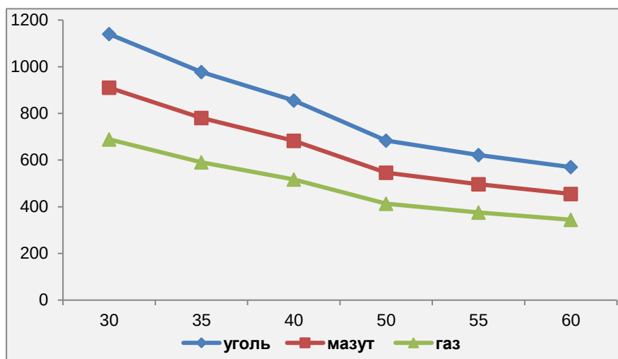
Рис. 1.35 - Выбросы CO 2 , г/кВт*ч в зависимости от КПД (нетто), %
