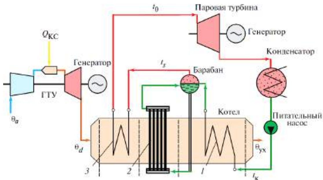
Рис. 3.12 - Схема простейшей утилизационной ПГУ КЭС с процессом генерации пара в котле-утилизаторе 1 — экономайзер; 2 — испаритель; 3 — пароперегреватель
