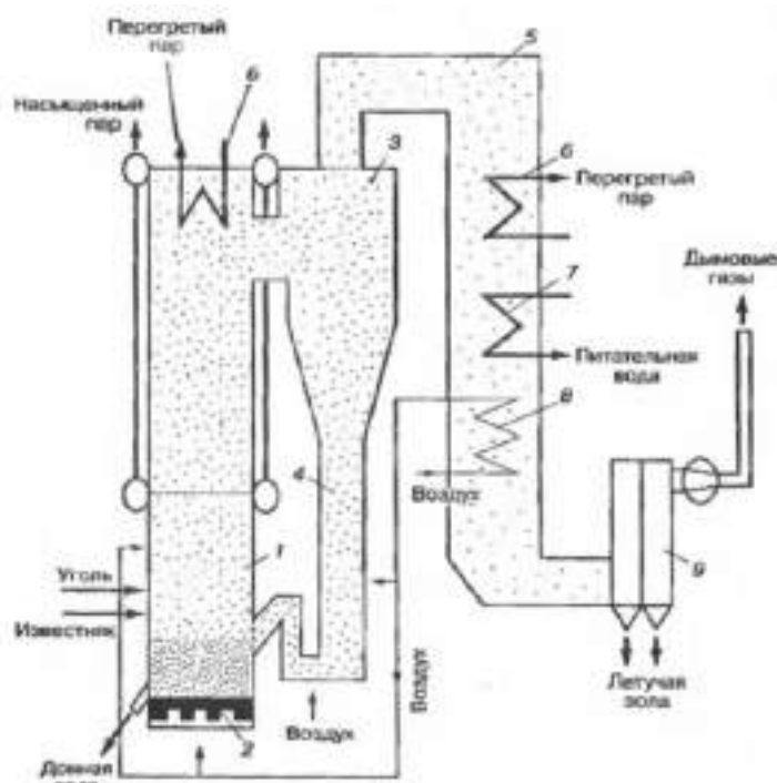
Рис. 5.7 - Принципиальная схема котла ЦКС системы «Пирофлоу»
