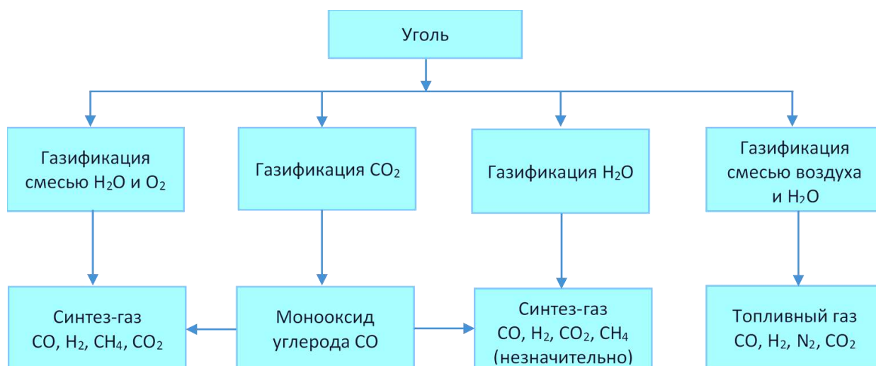
Рис. 3.14- Способы газификации угля
