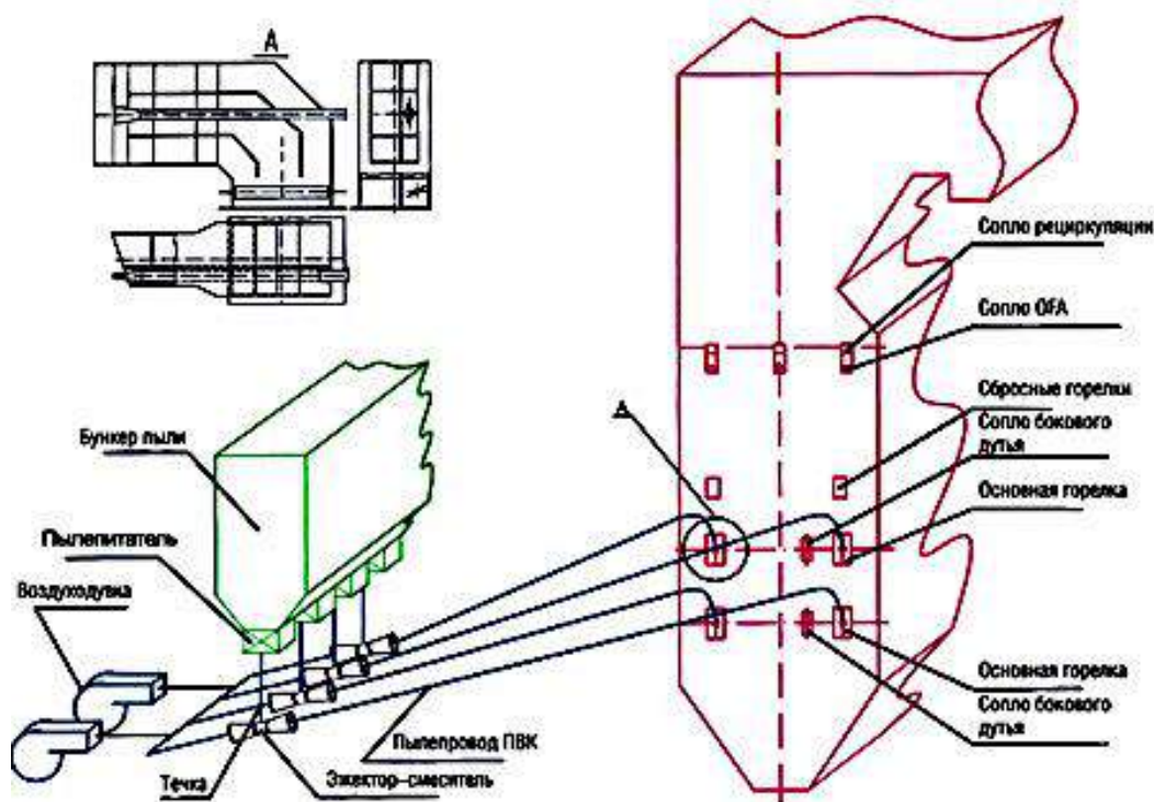
Рис. 4.27 - Схема подачи пыли высокой концентрации
