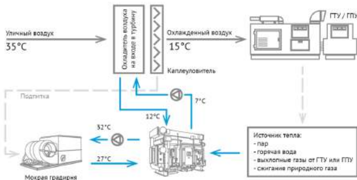
Рисунок 7.5 - Структурная схема АБХМ
