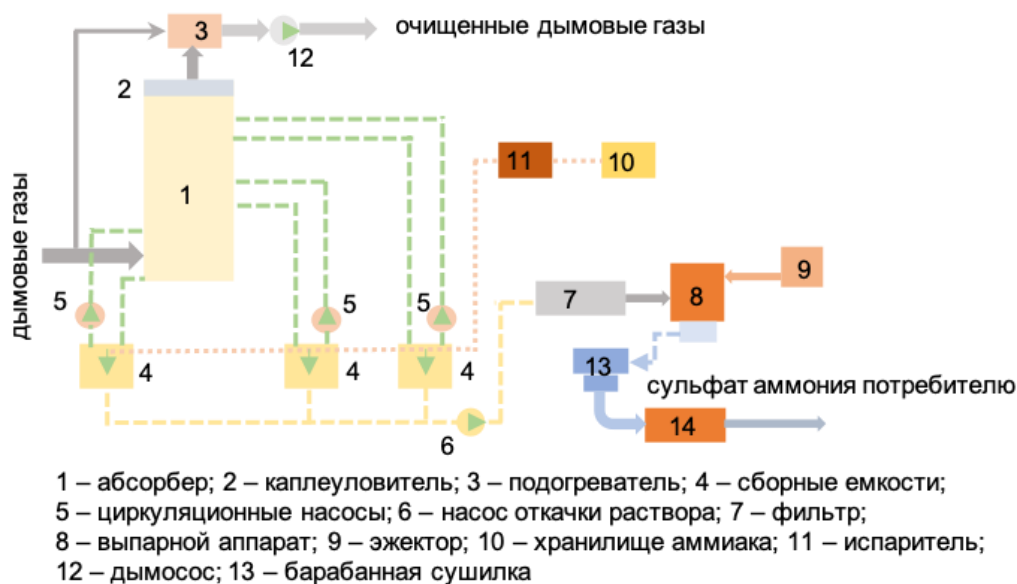
Рис.5.43 – Схема аммиачно-сульфатной сероочистки
