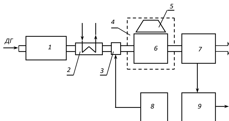
Рис. 4.37 – Принципиальная технологическая схема установки электронно-лучевой очистки дымовых газов ТЭС от оксидов серы и азота: ДГ – дымовые газы; 1 – электрофильтр; 2 – теплообменник; 3 – смеситель; 4 – радиационная защита; 5 – ускоритель электронов; 6 – реактор; 7 – фильтр; 8 – узел хранения, подготовки и подачи аммиака; 9 – гранулятор смеси сульфата и нитрата аммония
