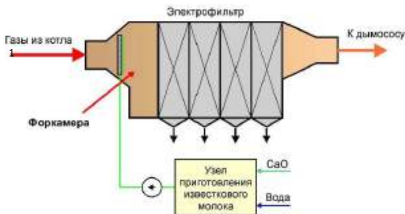
Рис. 4.13 Принципиальная схема упрощенной мокросухой известковой сероочистки [37]
