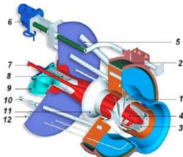
Рис. 4.21 – Горелка ФостерВиллер из серии Vortex
