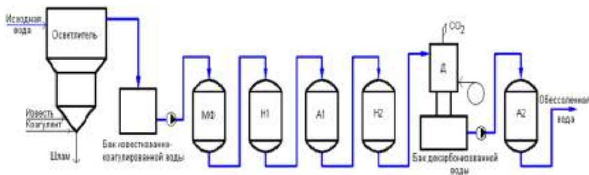
Рис. 4.39 - Схема химического обессоливания воды
