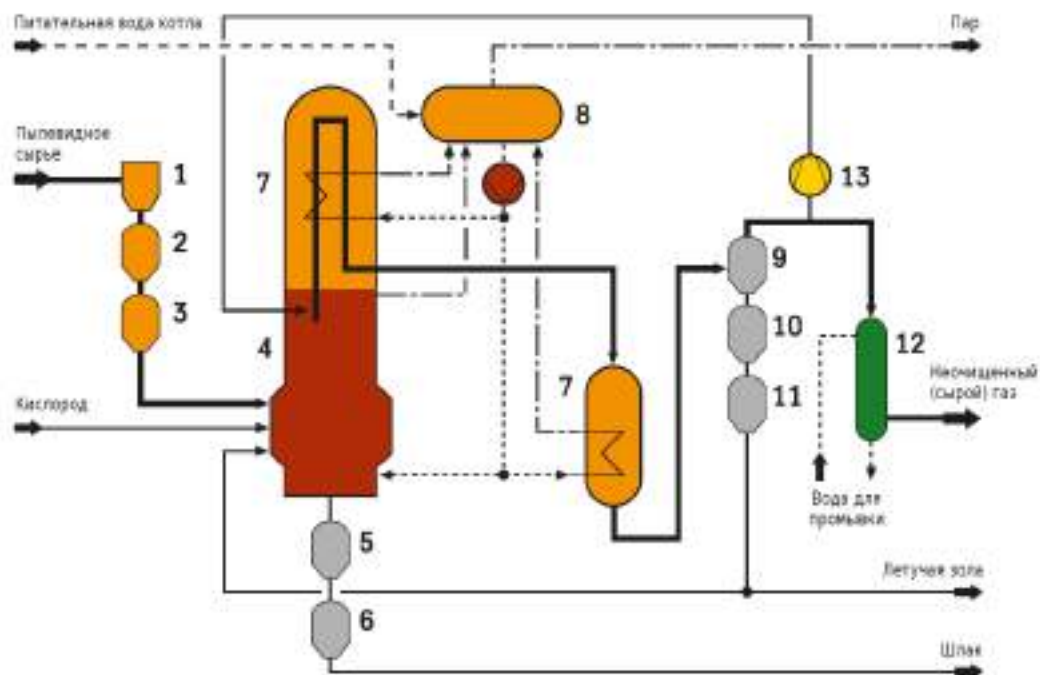
Рис. 3.16 - Технологическая схема технологии PRENFLO® PSG
