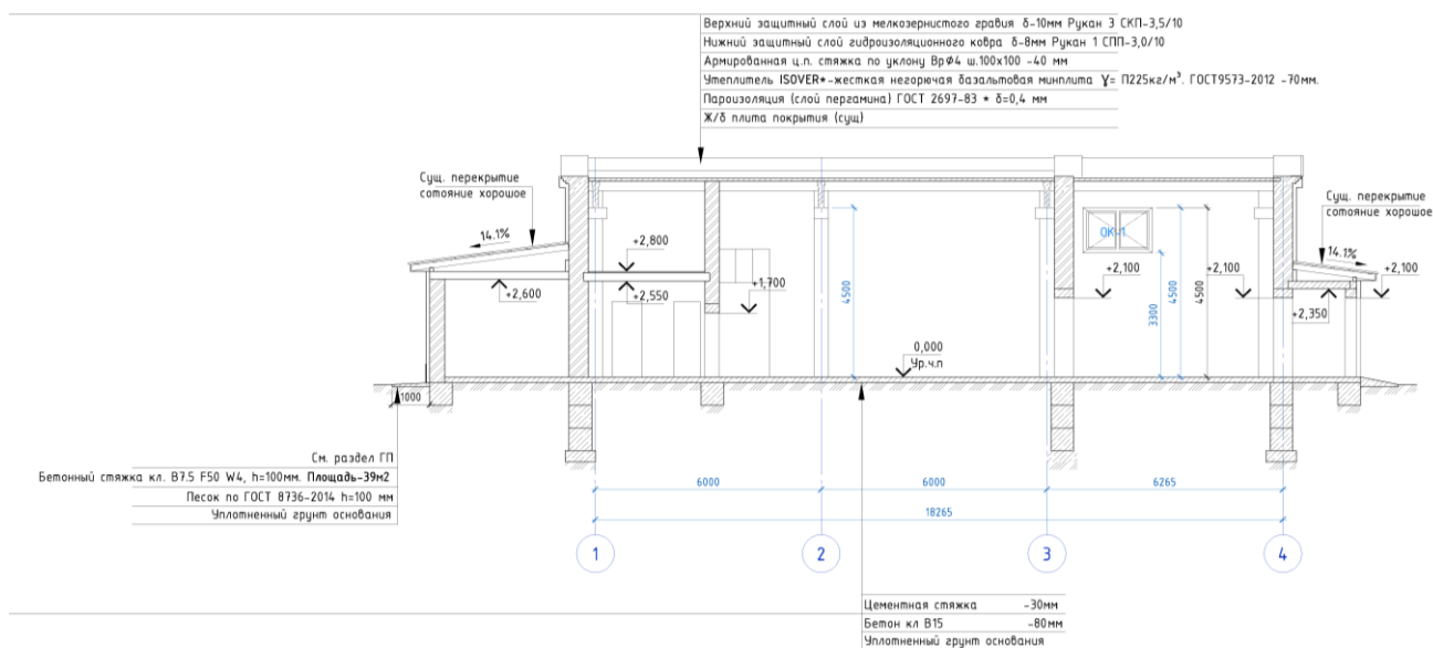
Разрез 2-2
