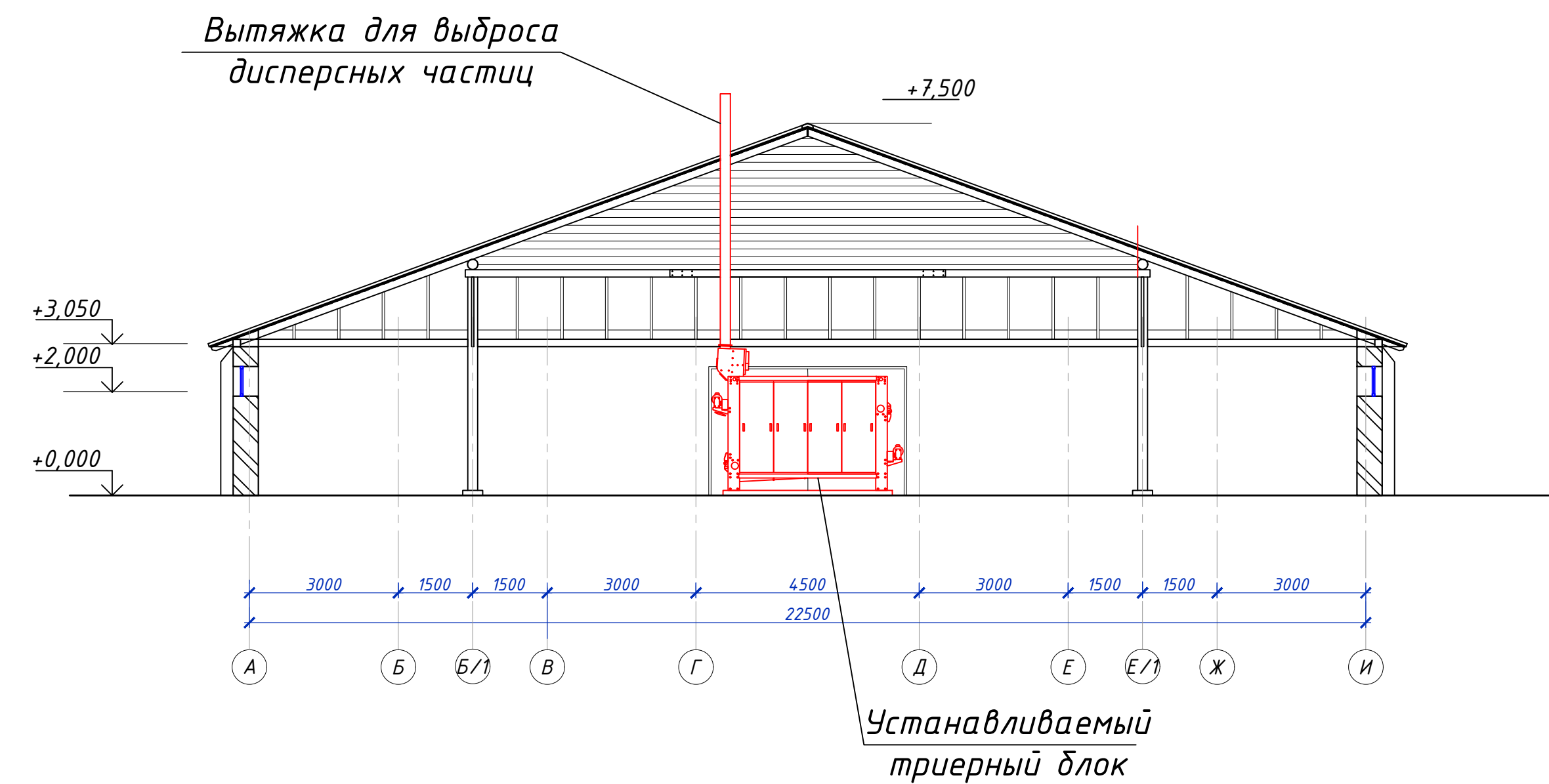
Разрез 2-2
